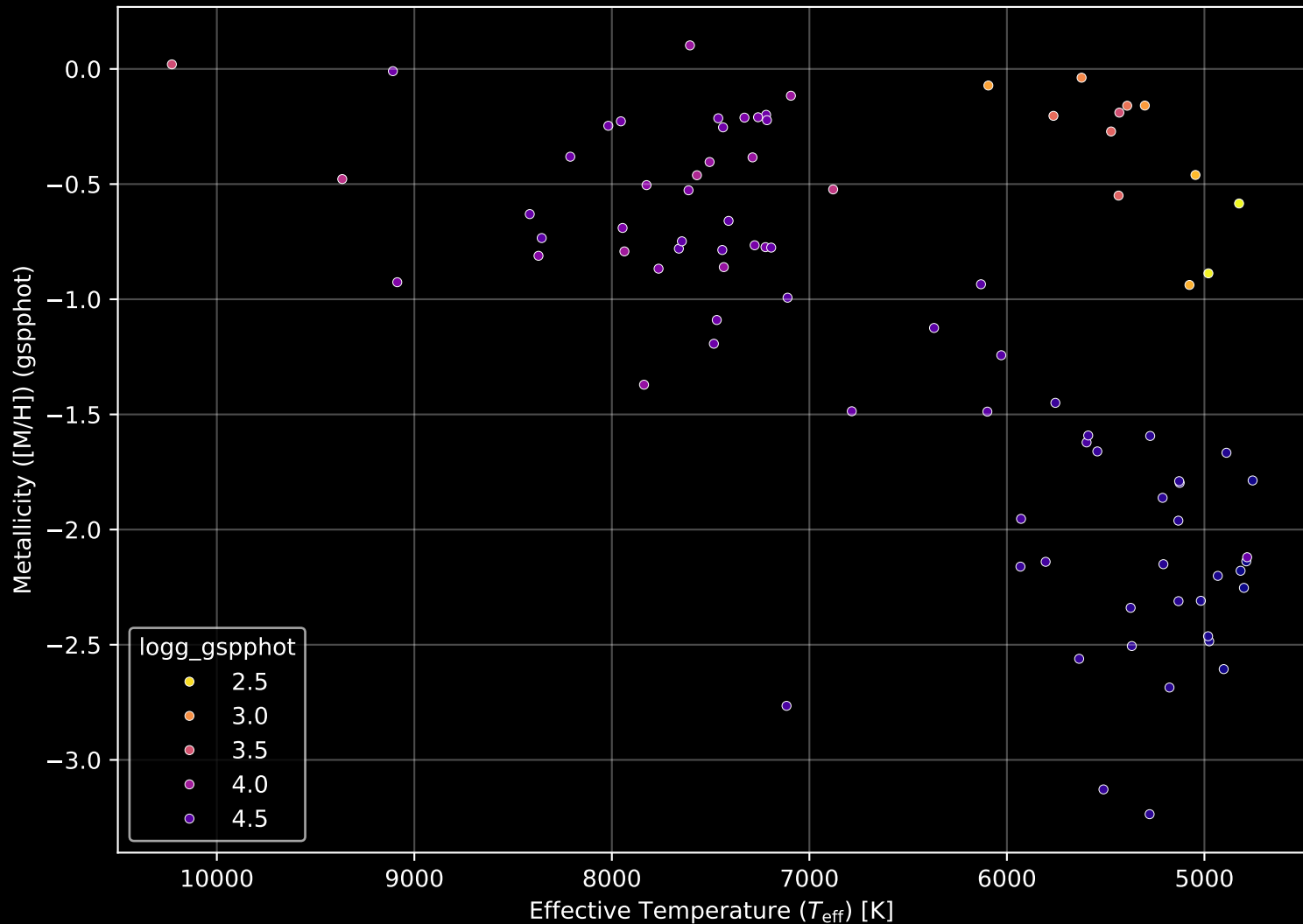
Gaia Cluster: [Ruprecht_75] Stellar Population Parameters (n= 88)
