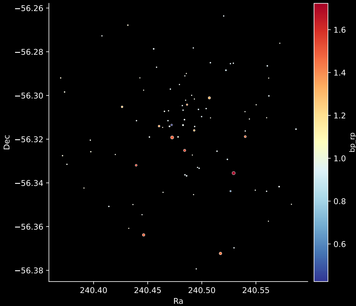
Gaia Cluster: [Ruprecht_75] Stars: 88
