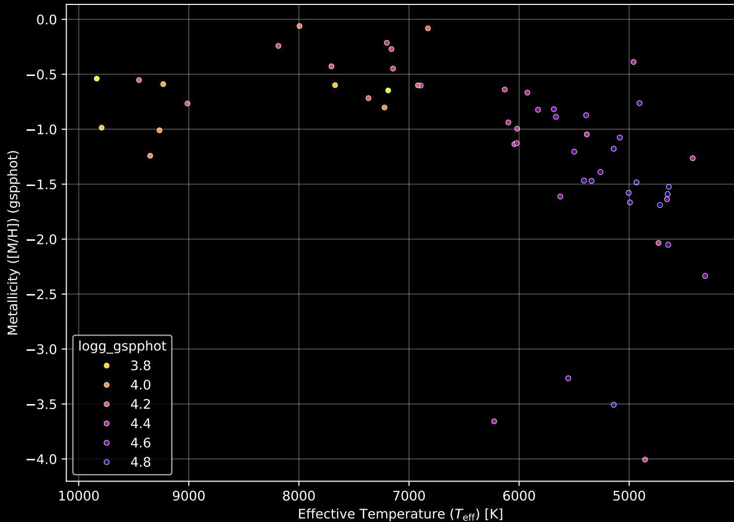
Gaia Cluster: [Ruprecht_76] Stellar Population Parameters (n= 55)
