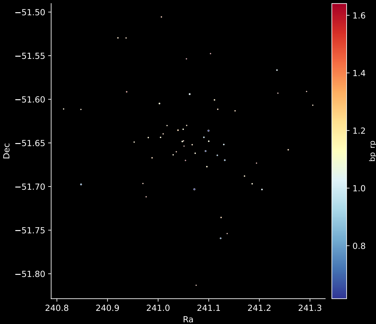
Gaia Cluster: [Ruprecht_76] Stars: 55
