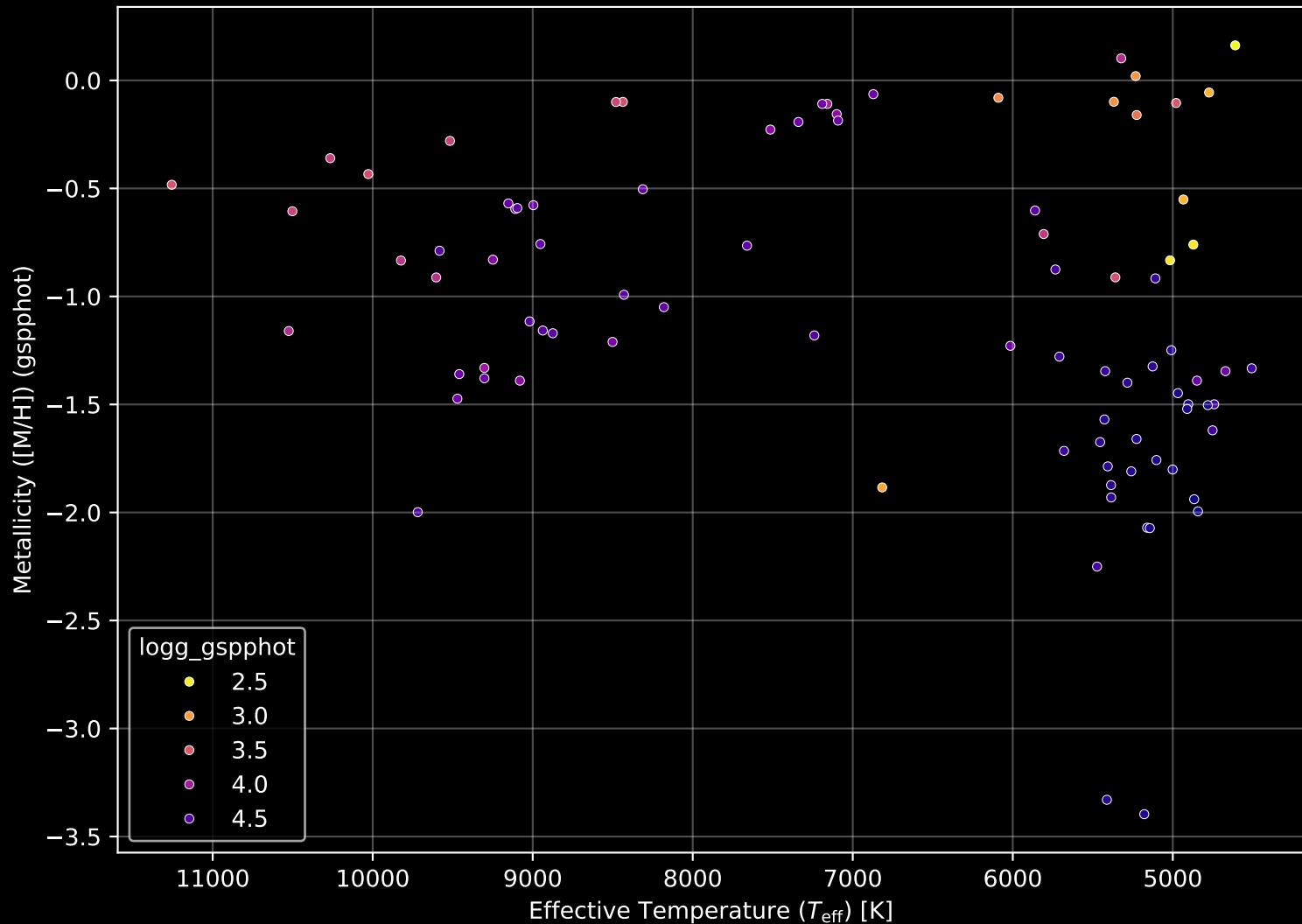
Gaia Cluster: [Ruprecht_77] Stellar Population Parameters (n= 88)
