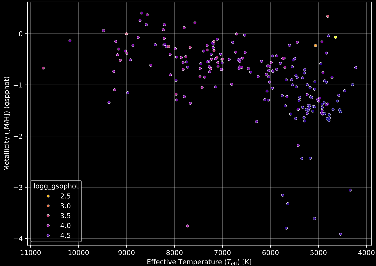
Gaia Cluster: [Ruprecht_82] Stellar Population Parameters (n= 208)
