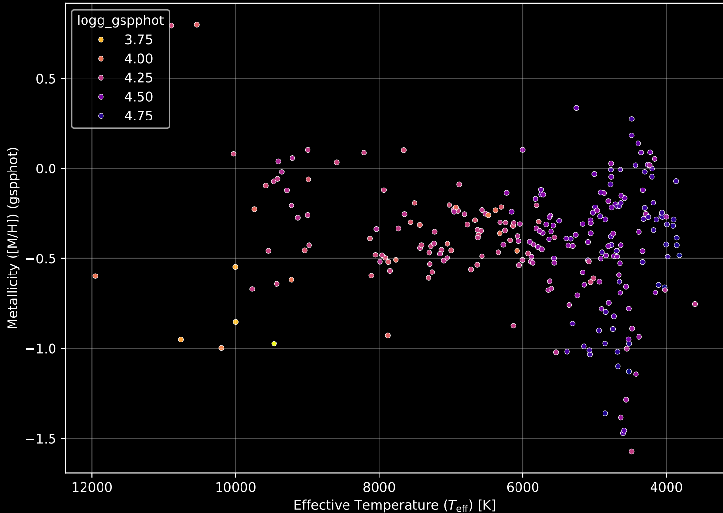
Gaia Cluster: [Ruprecht_91] Stellar Population Parameters (n= 262)
