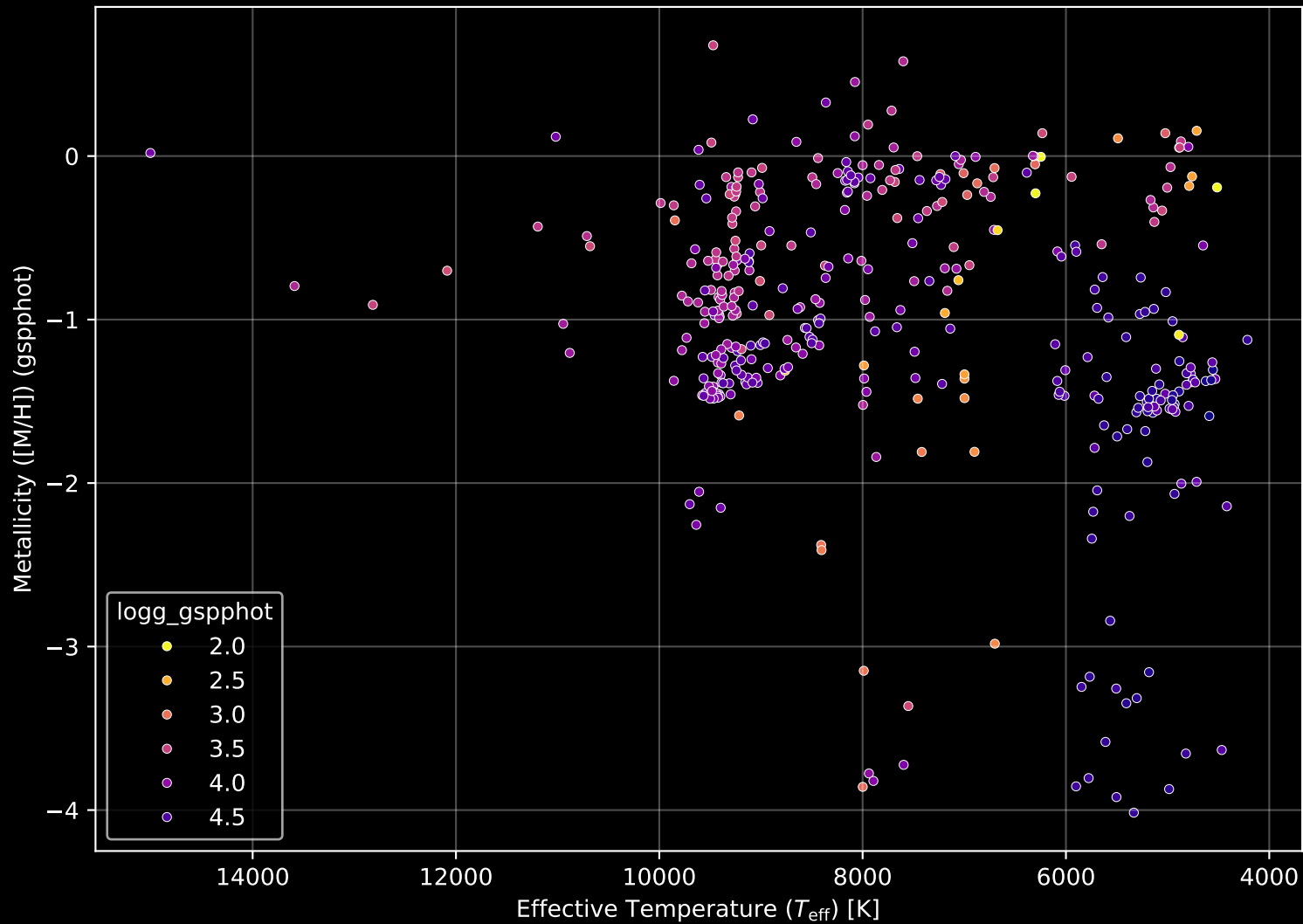
Gaia Cluster: [SAI_108] Stellar Population Parameters (n= 402)
