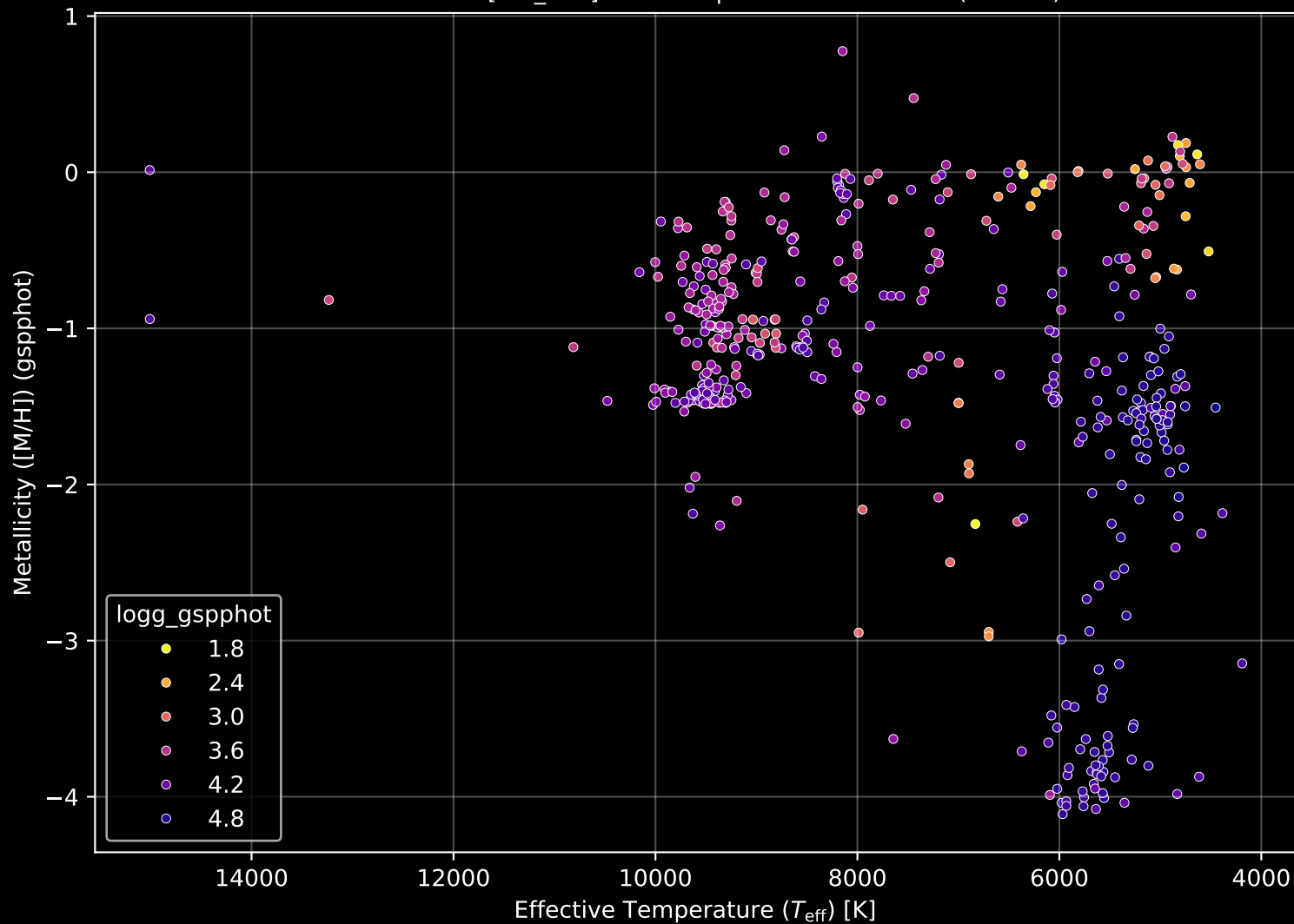
Gaia Cluster: [SAI_116] Stellar Population Parameters (n= 472)
