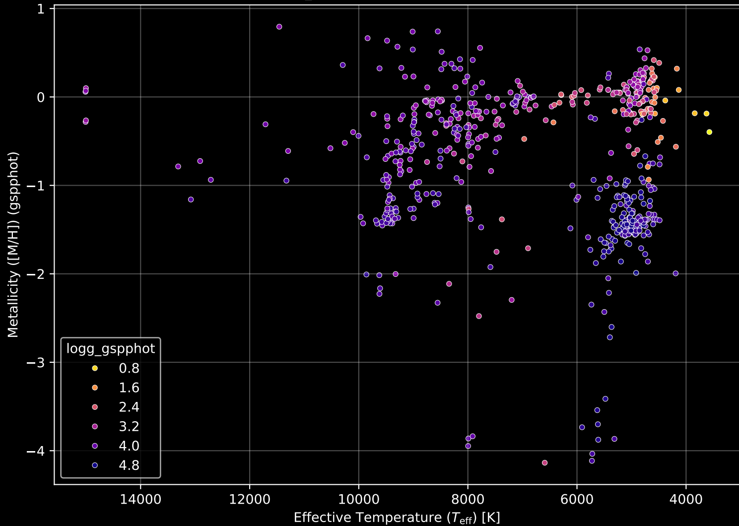
Gaia Cluster: [SAI_132] Stellar Population Parameters (n= 599)
