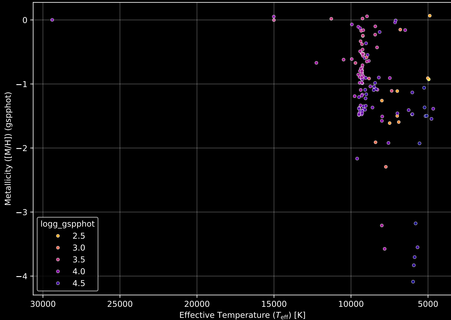
Gaia Cluster: [SAI_149] Stellar Population Parameters (n= 131)
