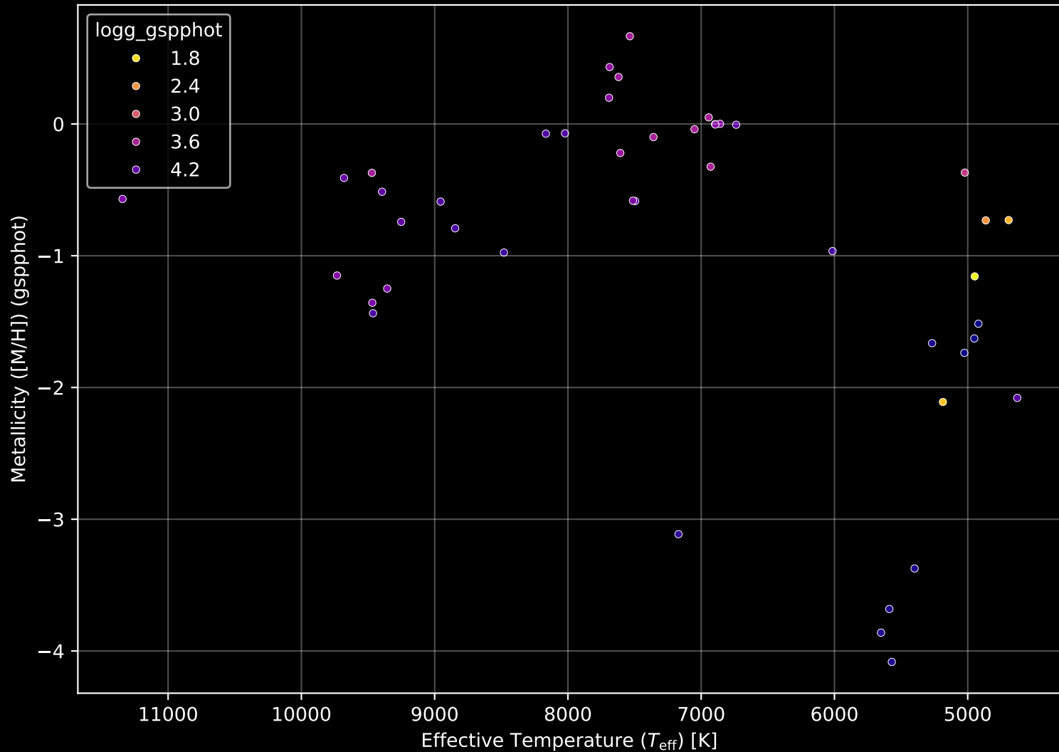
Gaia Cluster: [SAI_17] Stellar Population Parameters (n= 45)
