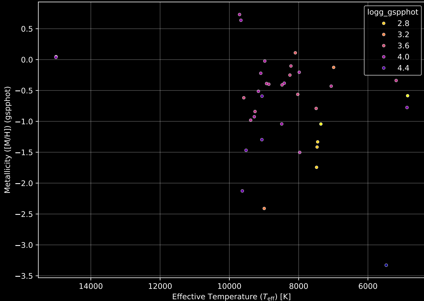
Gaia Cluster: [Saurer_2] Stellar Population Parameters (n= 39)
