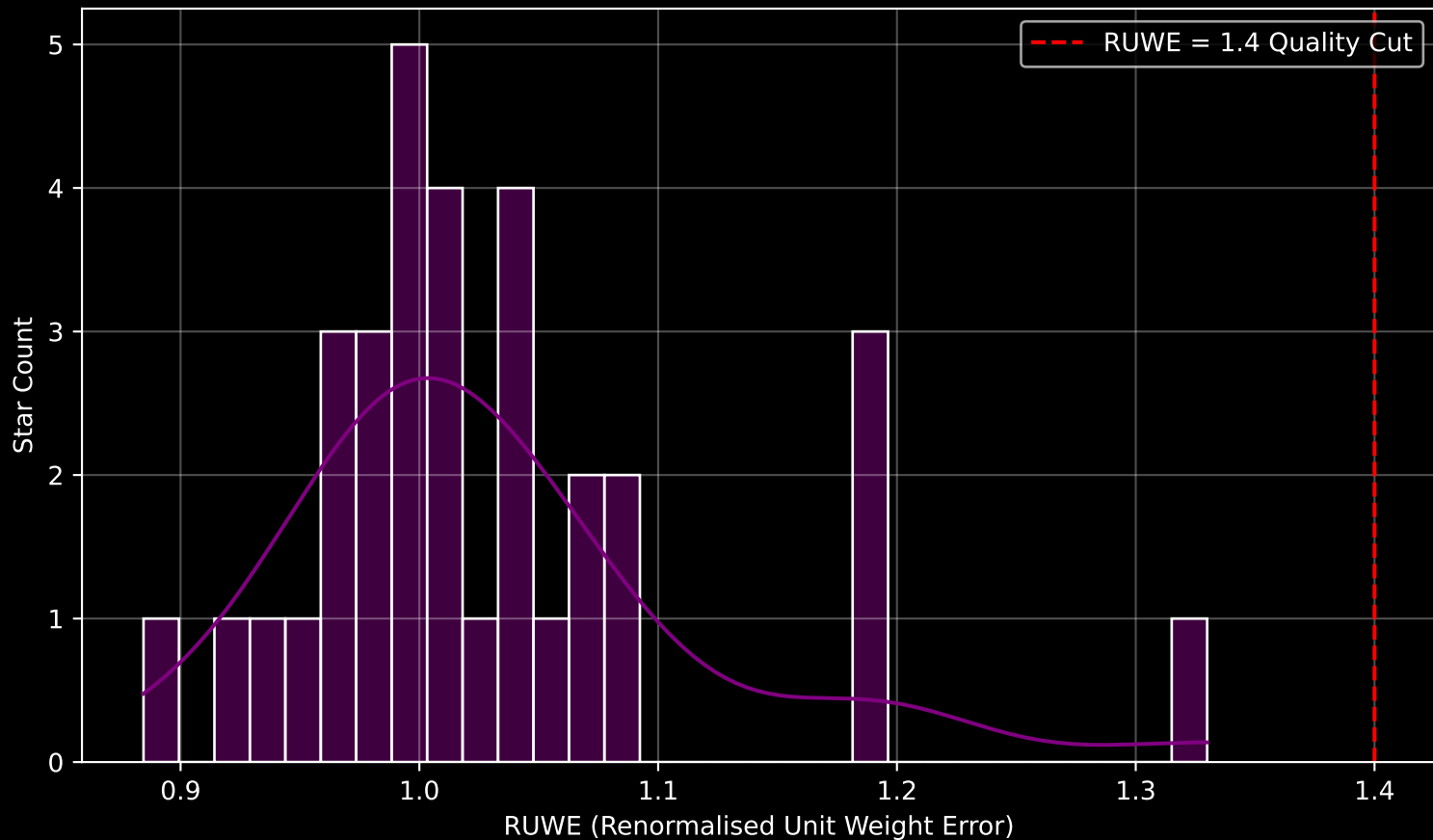
Gaia Cluster: [Sher_1] RUWE Distribution (n= 33)
