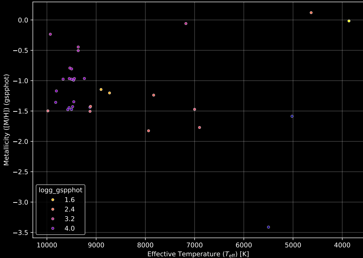
Gaia Cluster: [Sher_1] Stellar Population Parameters (n= 33)
