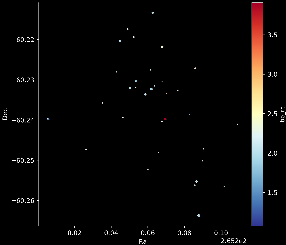
Gaia Cluster: [Sher_1] Stars: 33
