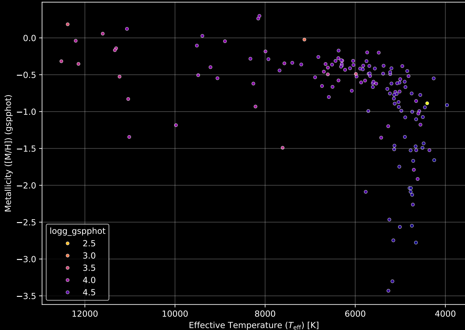
Gaia Cluster: [Stock_4] Stellar Population Parameters (n= 143)
