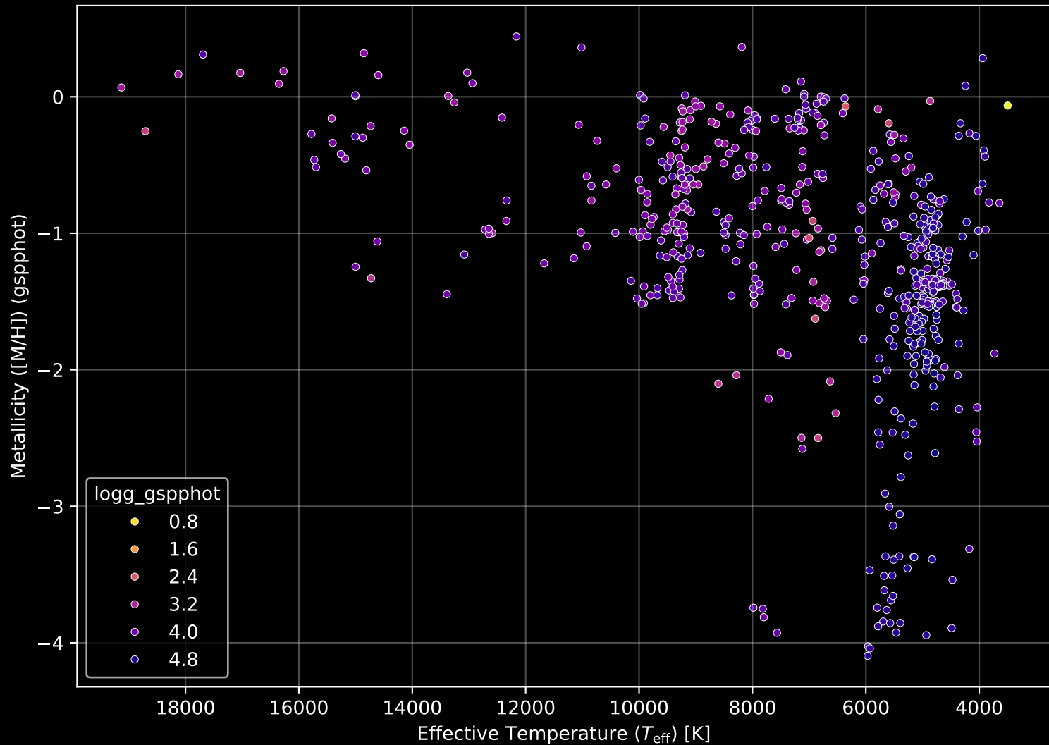
Gaia Cluster: [Stock_8] Stellar Population Parameters (n= 590)
