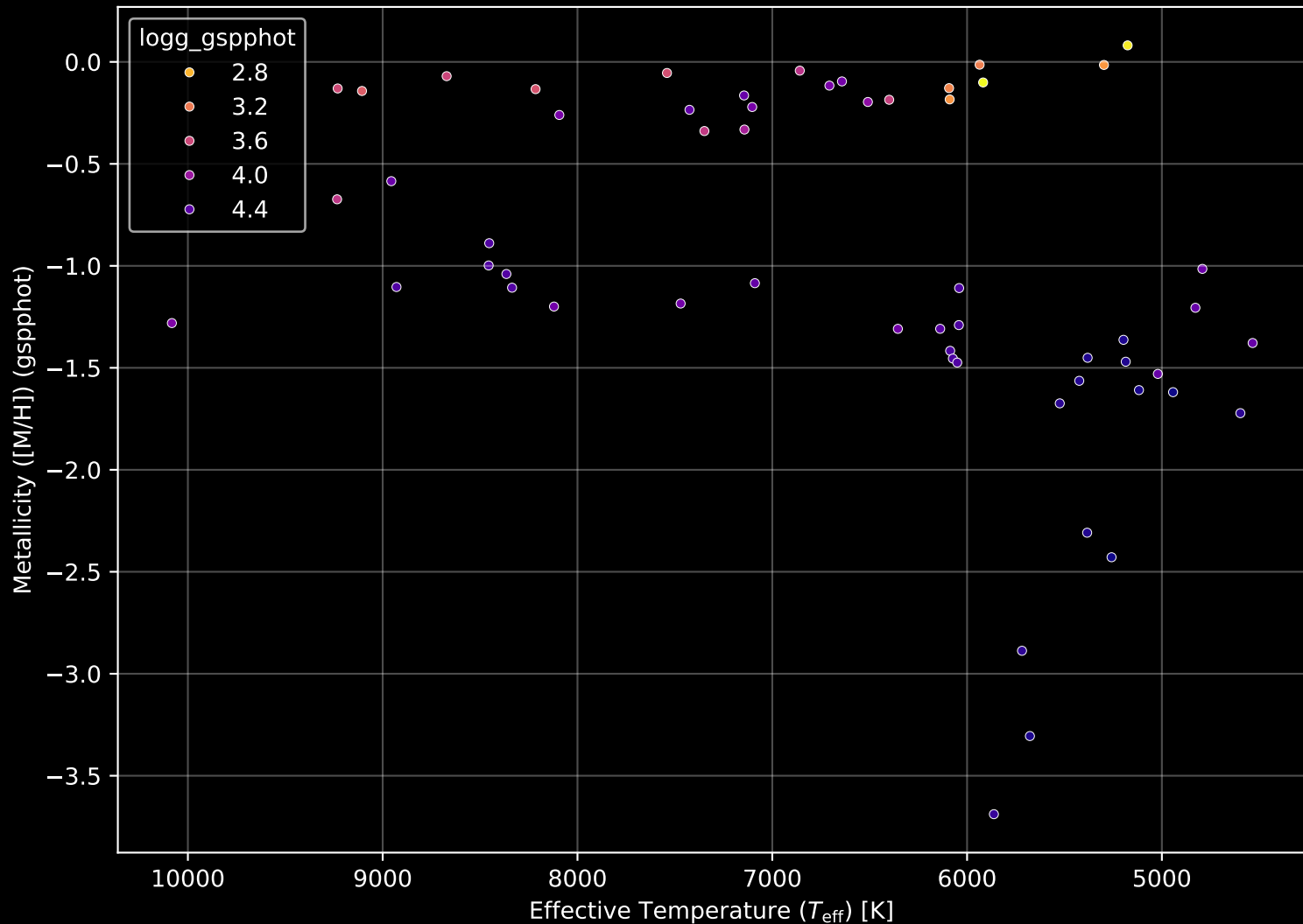
Gaia Cluster: [Teutsch_103] Stellar Population Parameters (n= 57)
