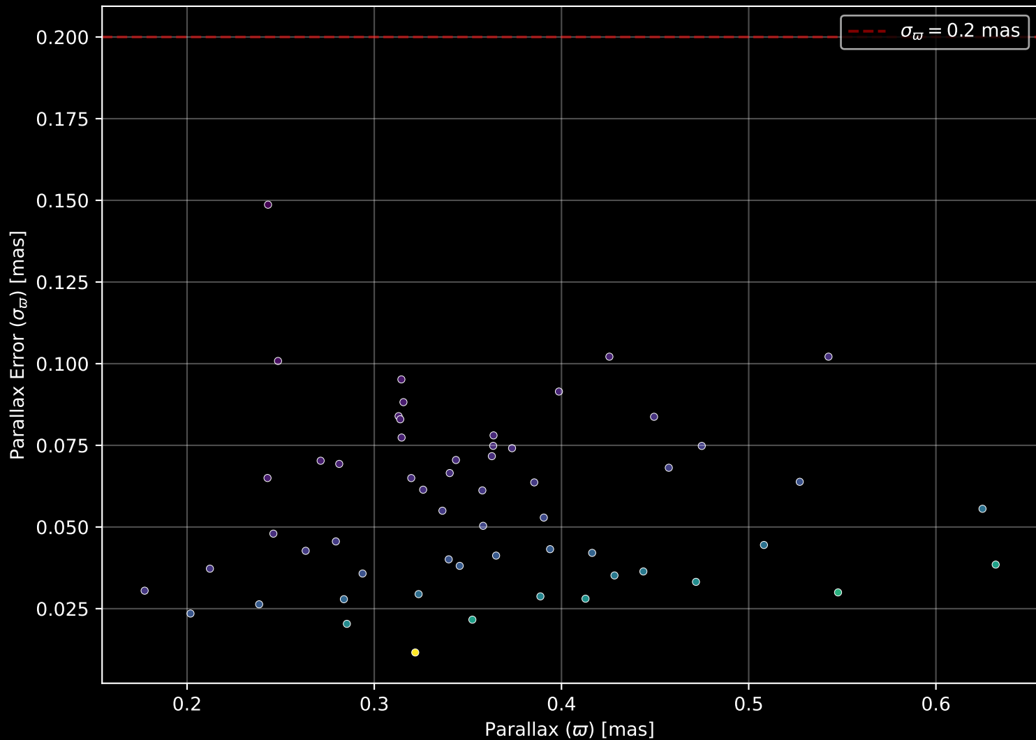
Gaia Cluster: [Deutsch 103] Parallax Quality (n= 57)
