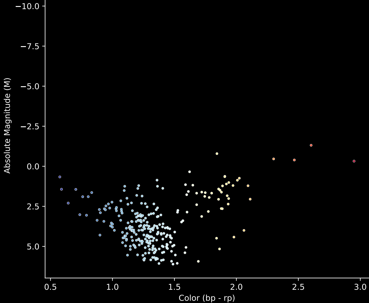
Gaia Cluster: [Deutsch_12] Stars (n= 273) Hertzprung-Russel Diagram
