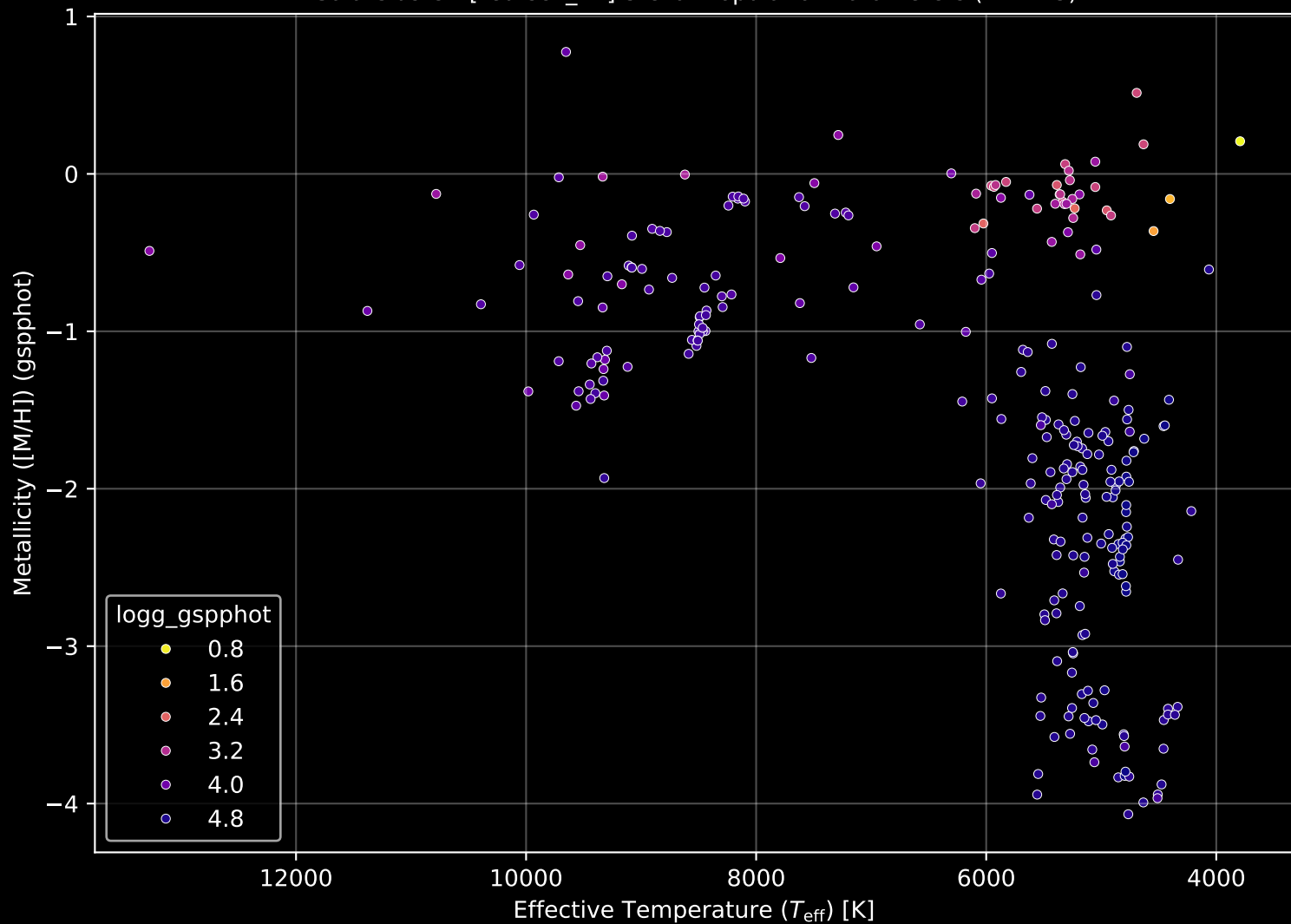
Gaia Cluster: [Deutsch_12] Stellar Population Parameters (n= 273)
