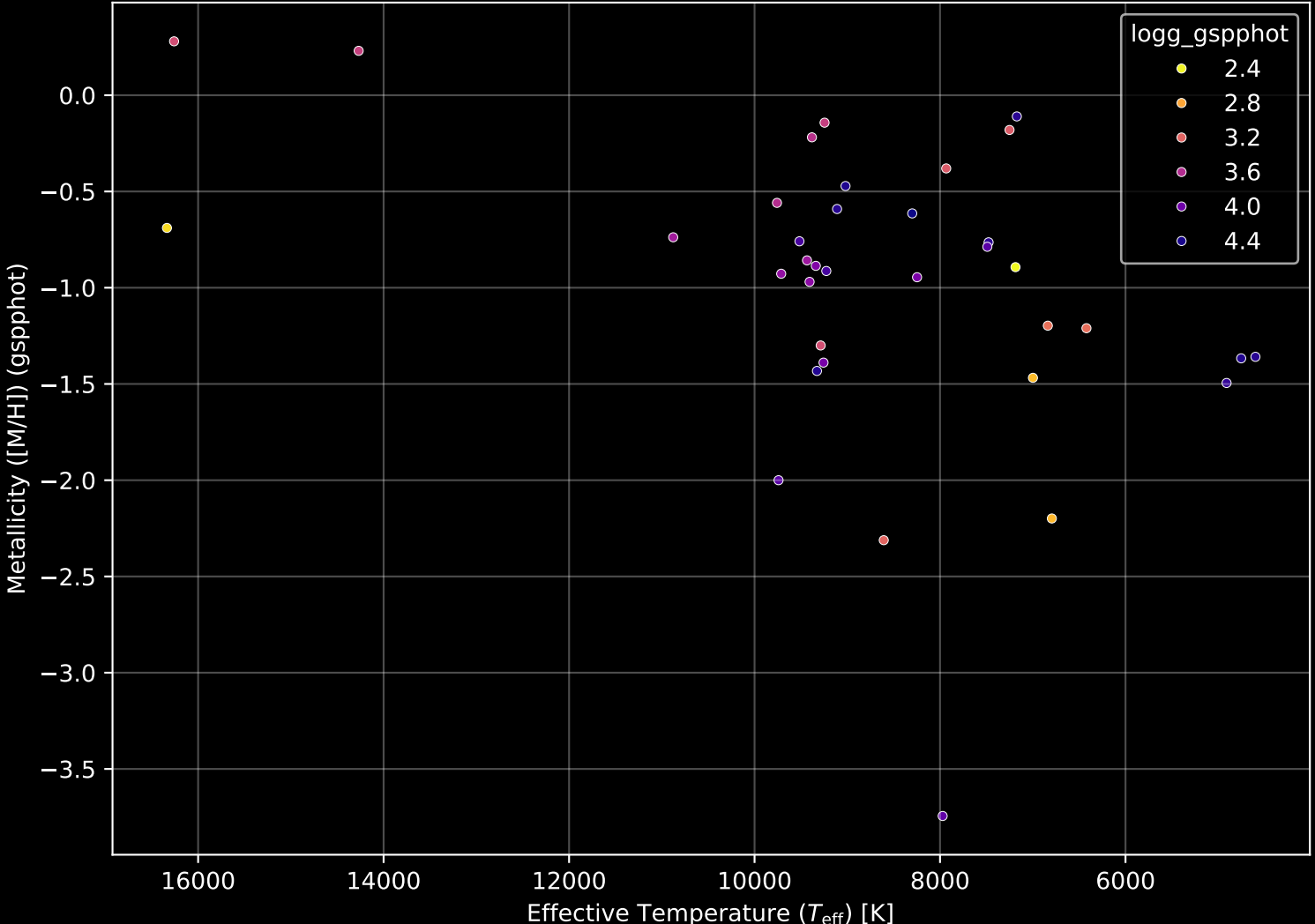
Gaia Cluster: [Deutsch 127] Stellar Population Parameters
