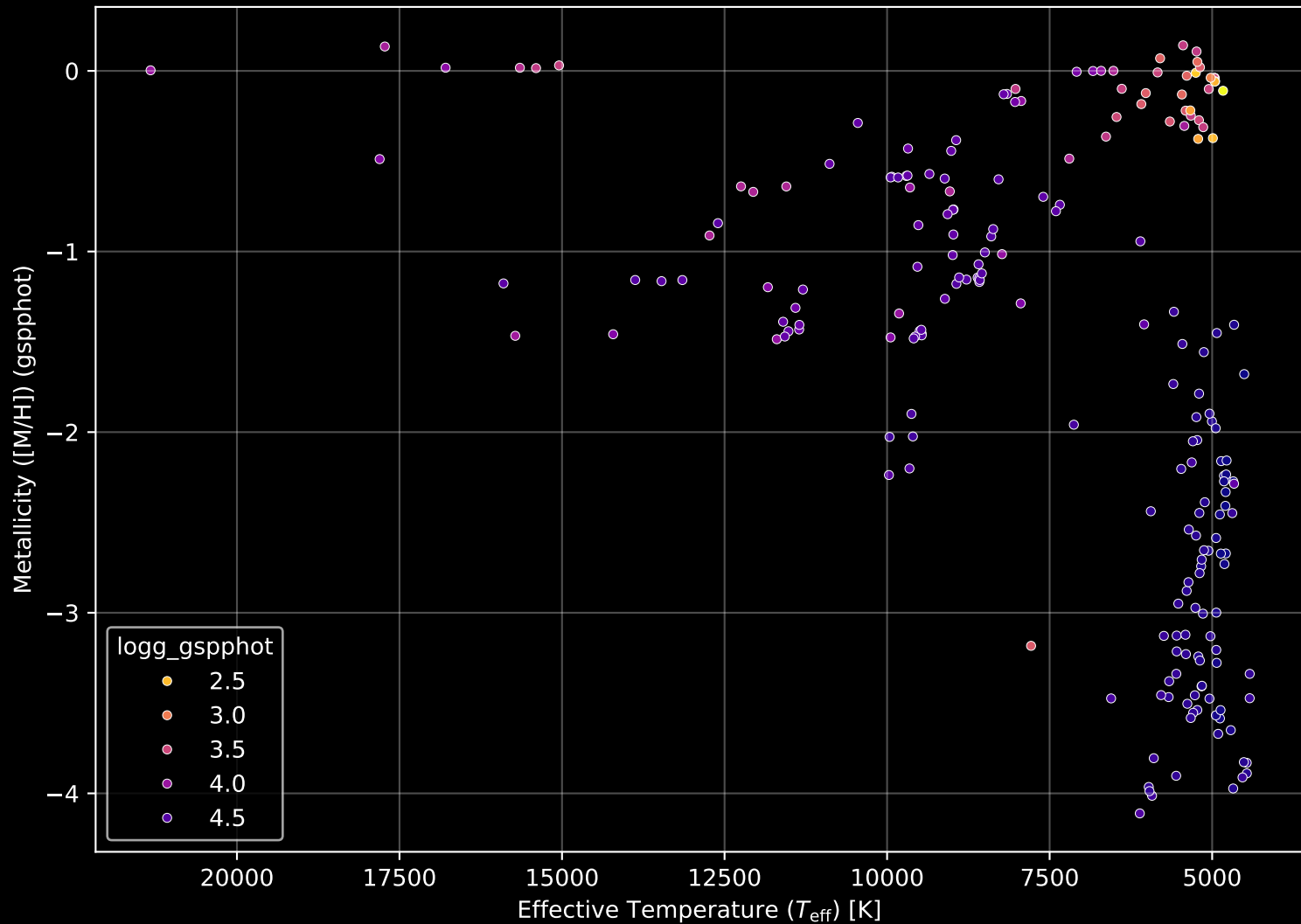
Gaia Cluster: [Teutsch_13] Stellar Population Parameters (n= 213)
