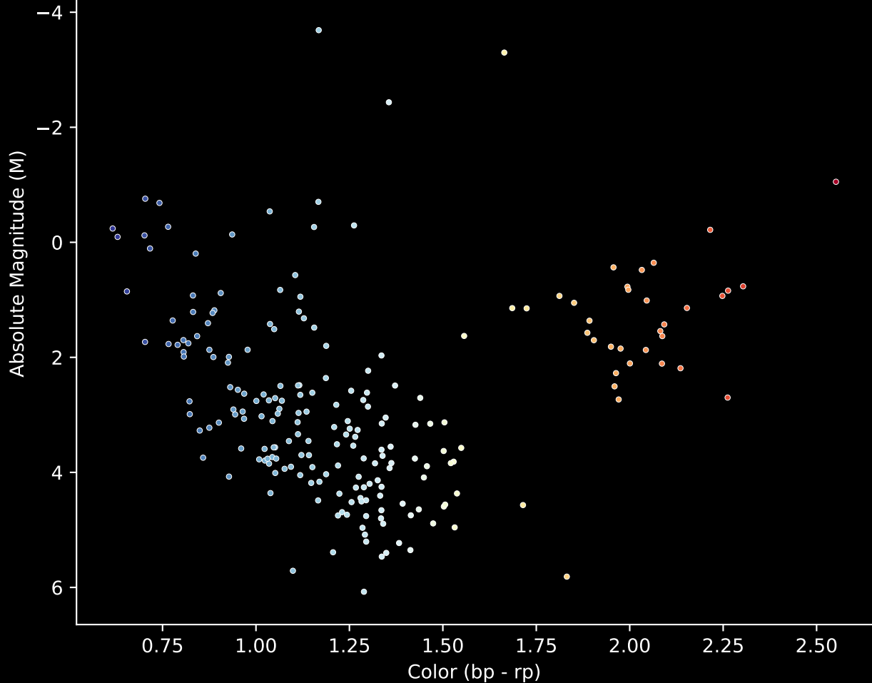
Gaia Cluster: [Deutsch_13] Stars (n= 213) Hertzsprung-Russel Diagram
