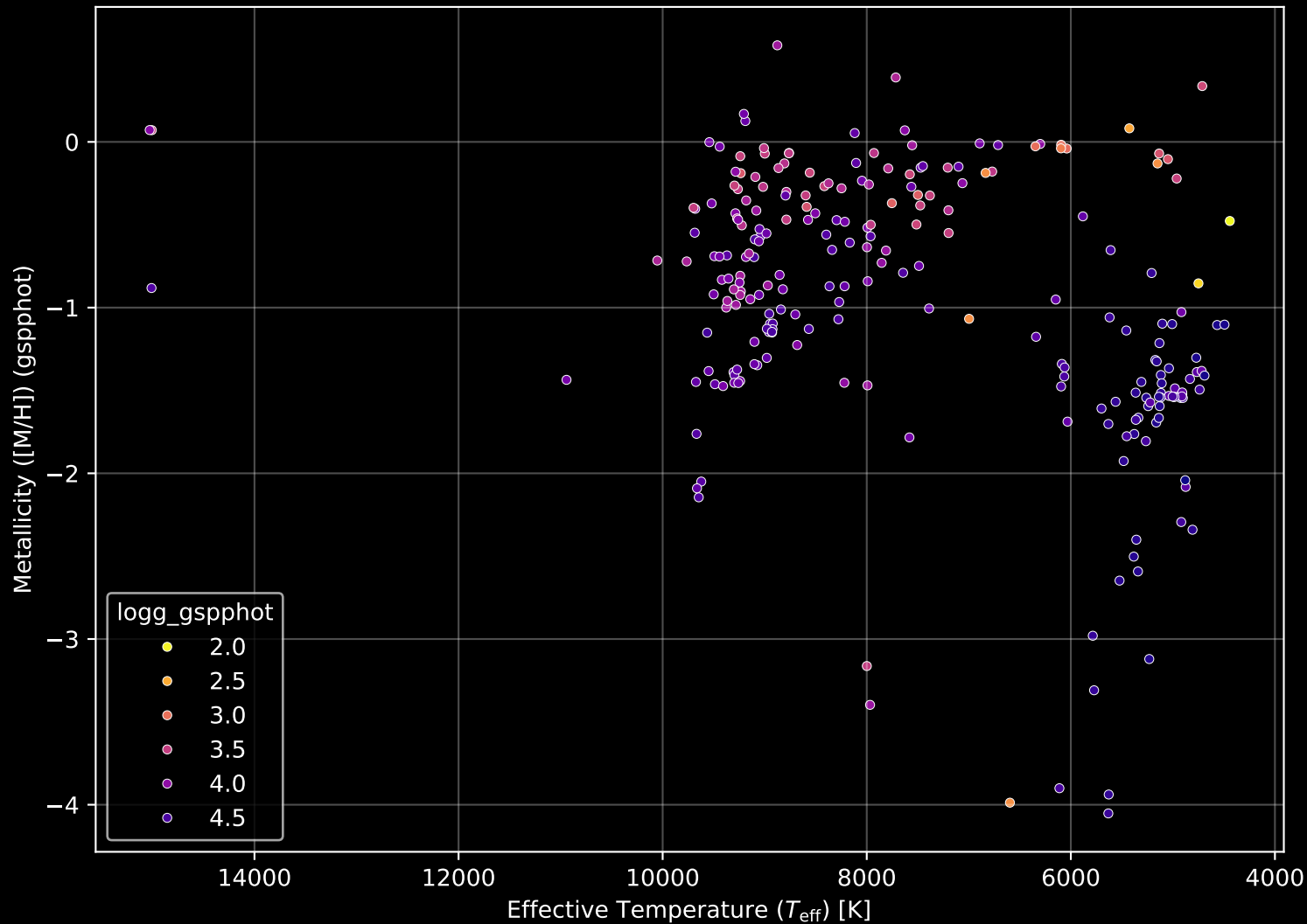
Gaia Cluster: [Teutsch_144] Stellar Population Parameters (n= 243)
