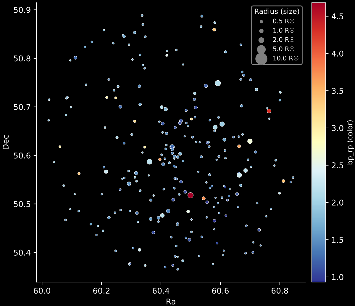
Gaia Cluster: [Deutsch_144] Stars: 243
