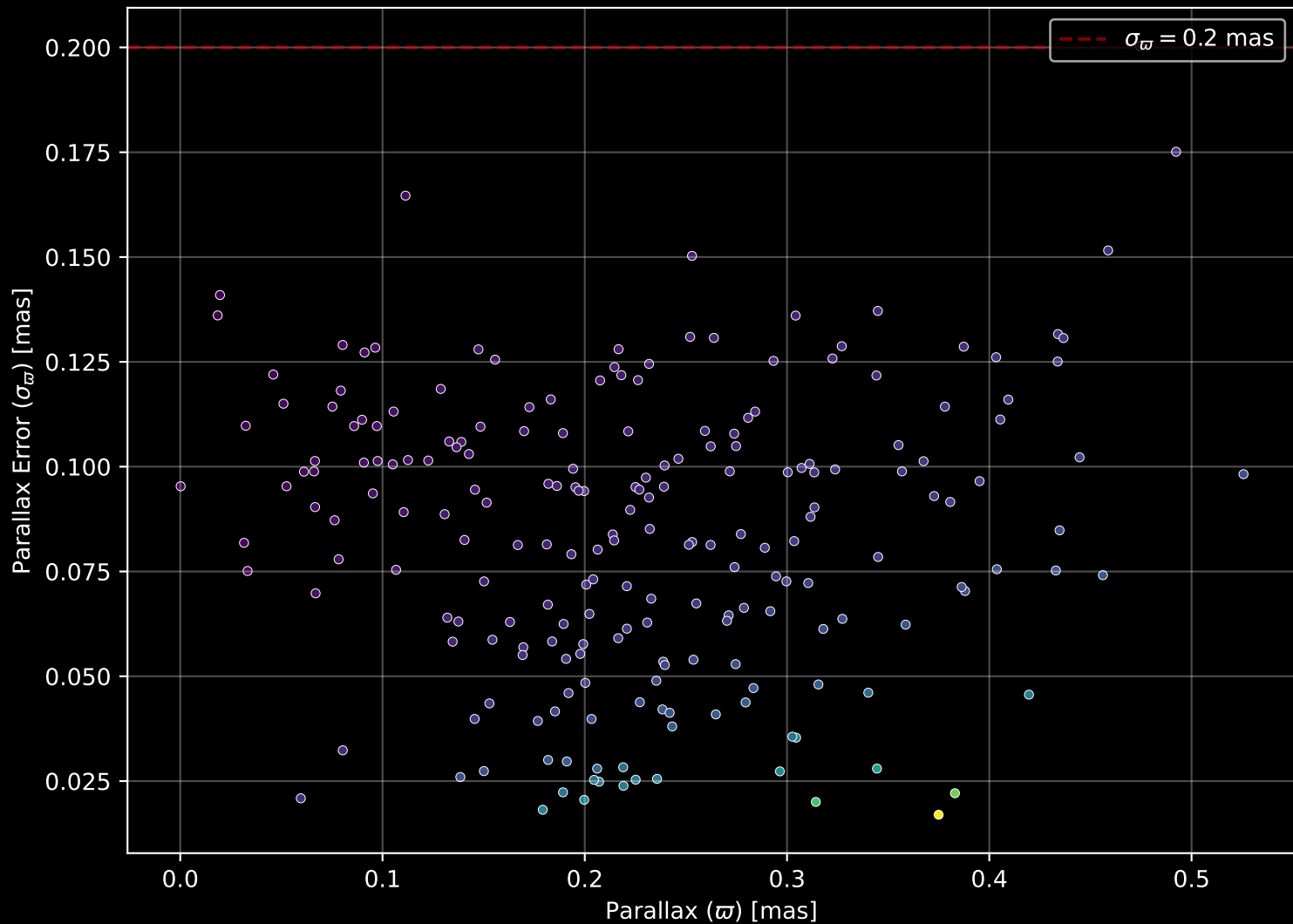
Gaia Cluster: [Deutsch_2] Parallax Quality (n= 212)
