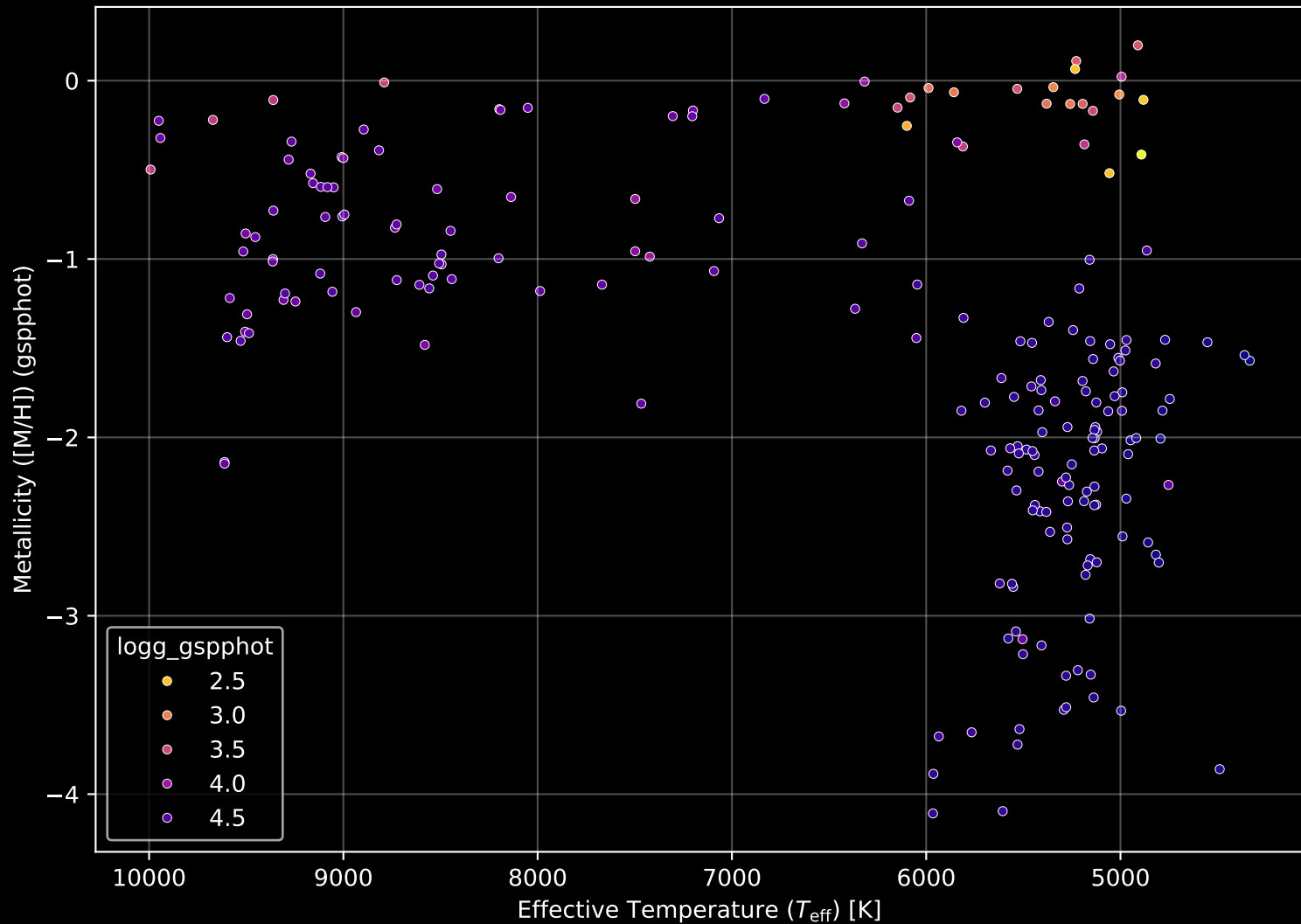
Gaia Cluster: [Teutsch_2] Stellar Population Parameters (n= 212)
