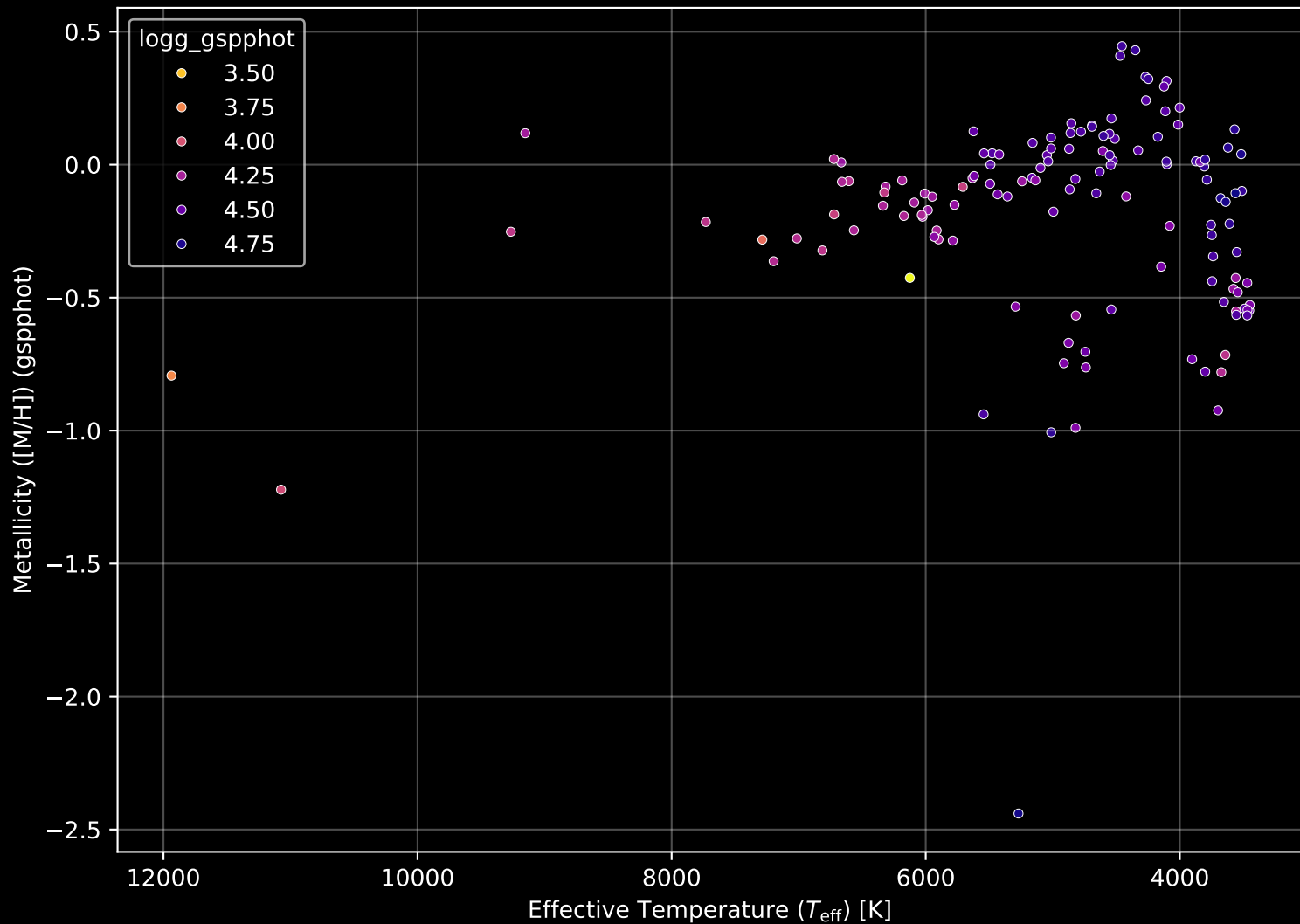
Gaia Cluster: [Teutsch_35] Stellar Population Parameters (n= 135)
