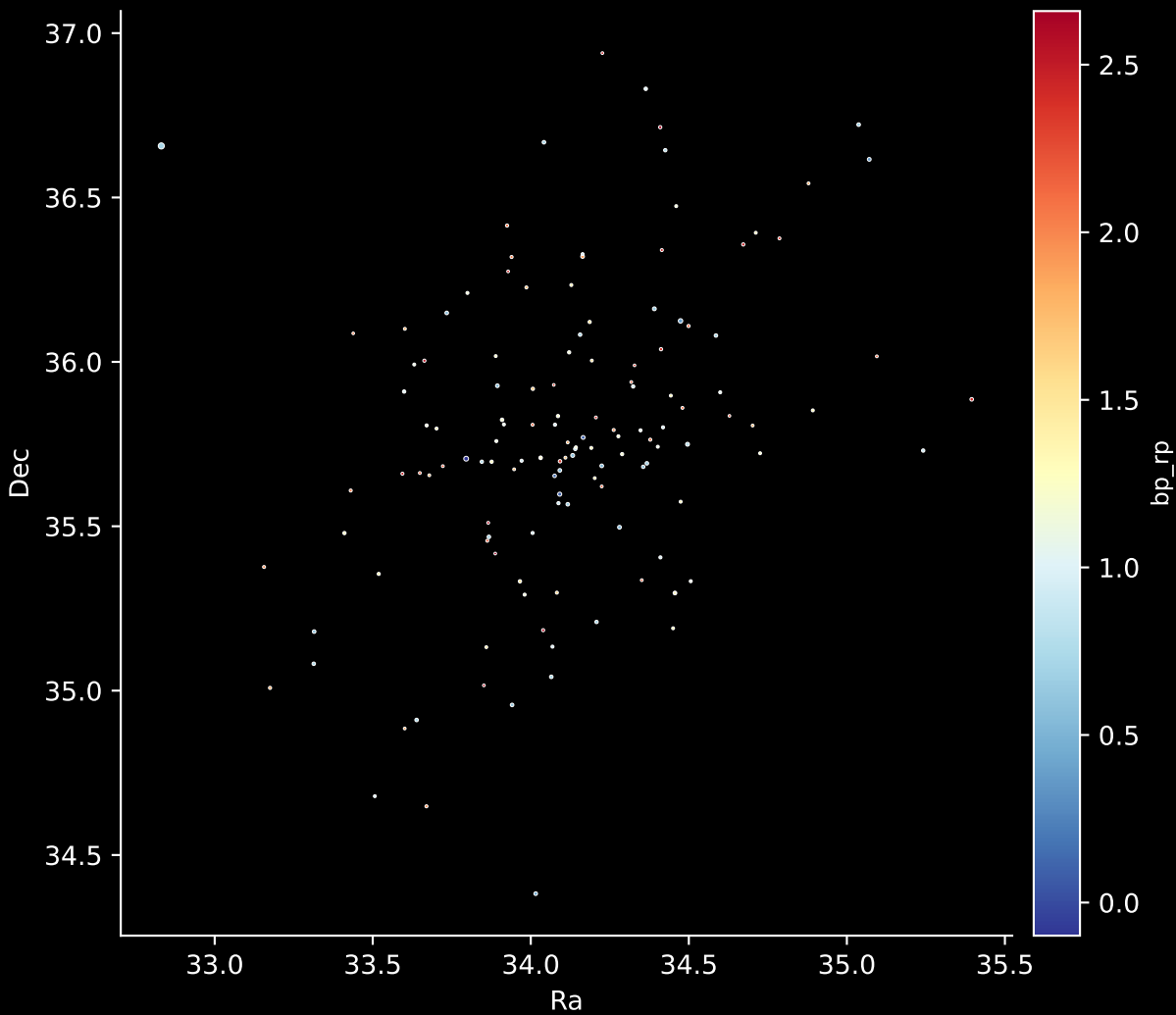
Gaia Cluster: [Teutsch_35] Stars: 135
