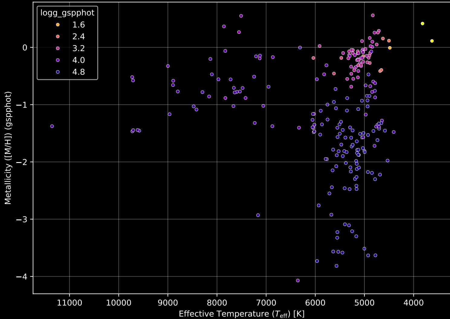
Gaia Cluster: [Deutsch_44] Stellar Population Parameters (n= 233)
