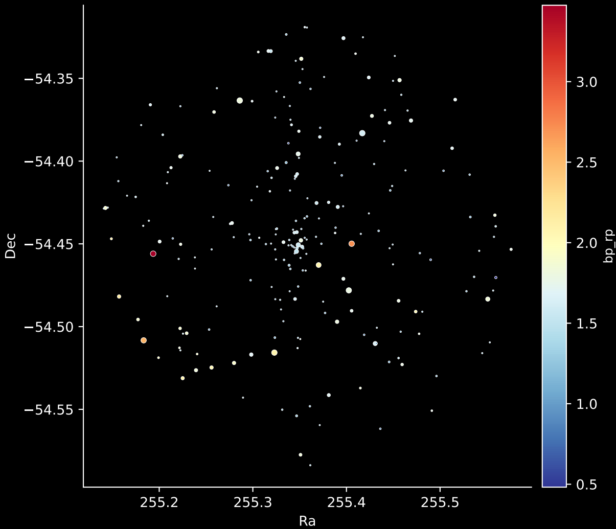
Gaia Cluster: [Deutsch_44] Stars: 233
