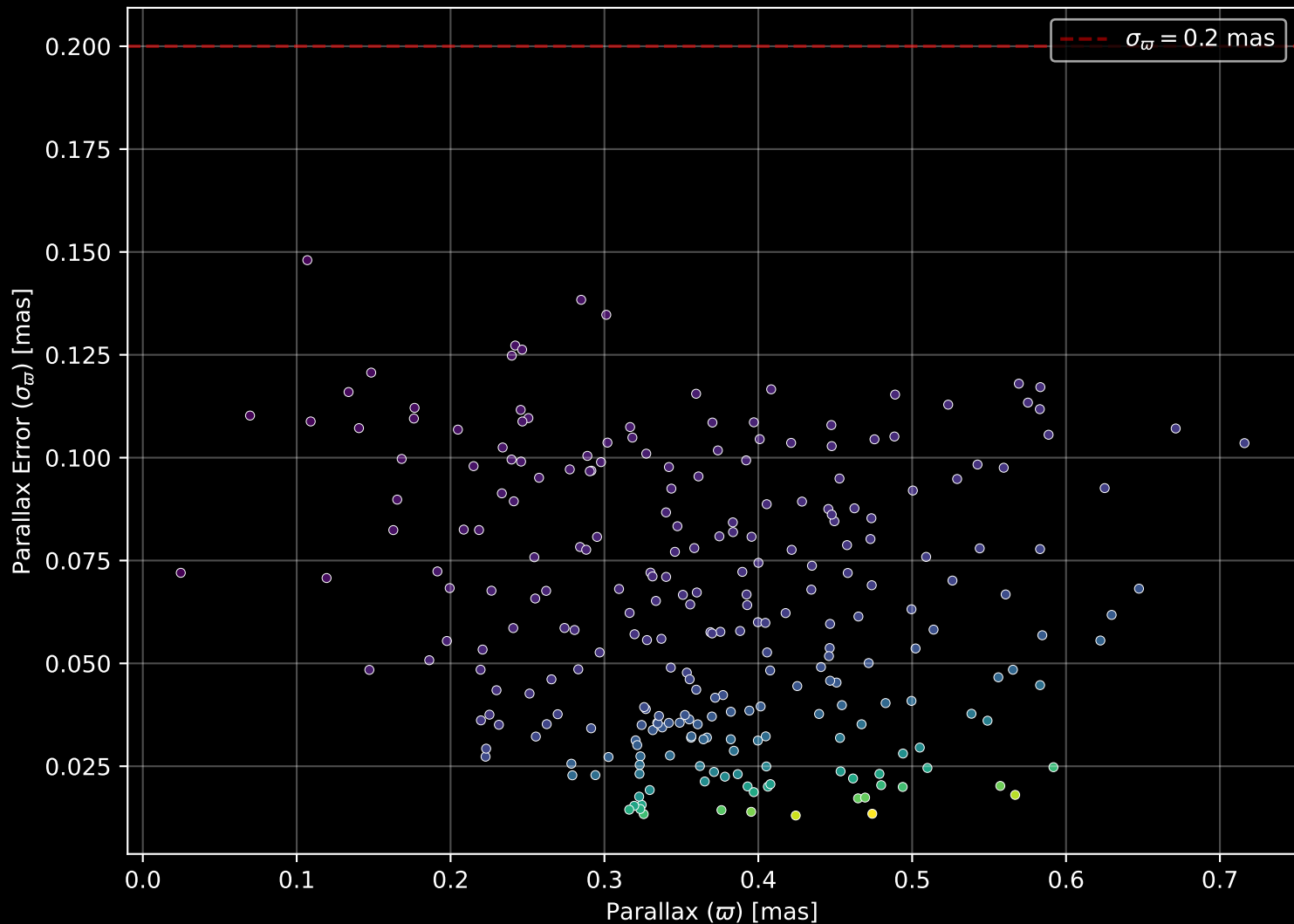
Gaia Cluster: [Deutsch_49] Parallax Quality (n= 255)
