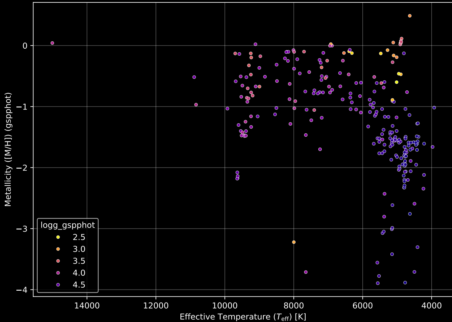
Gaia Cluster: [Deutsch_49] Stellar Population Parameters (n= 255)
