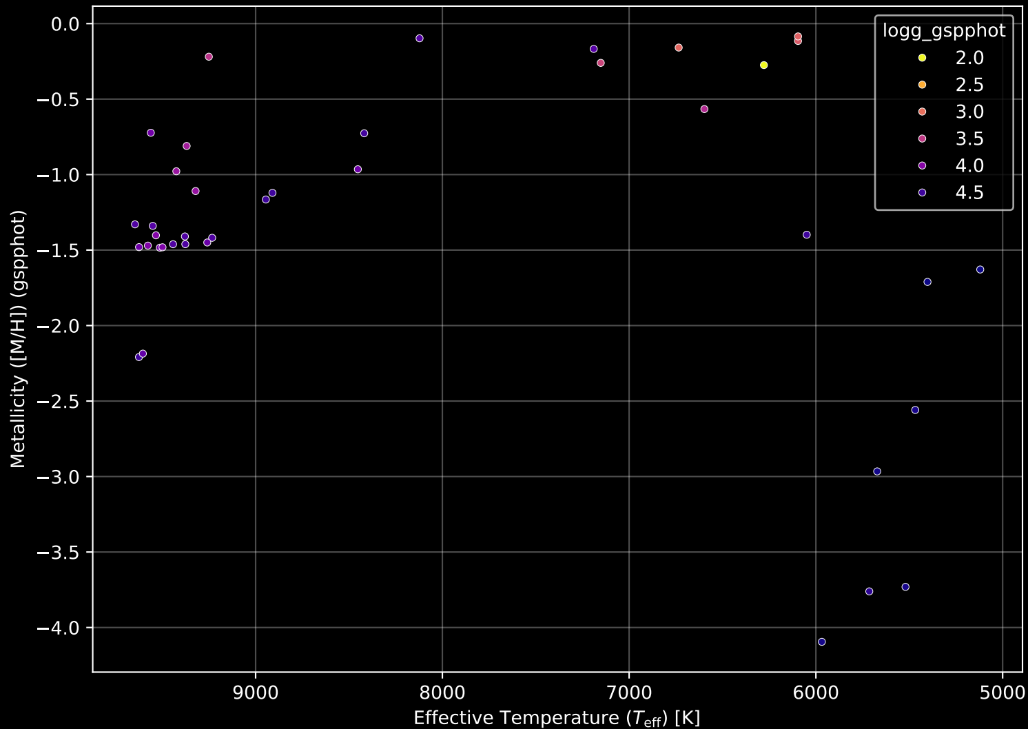
Gaia Cluster: [Deutsch_50] Stellar Population Parameters (n= 39)
