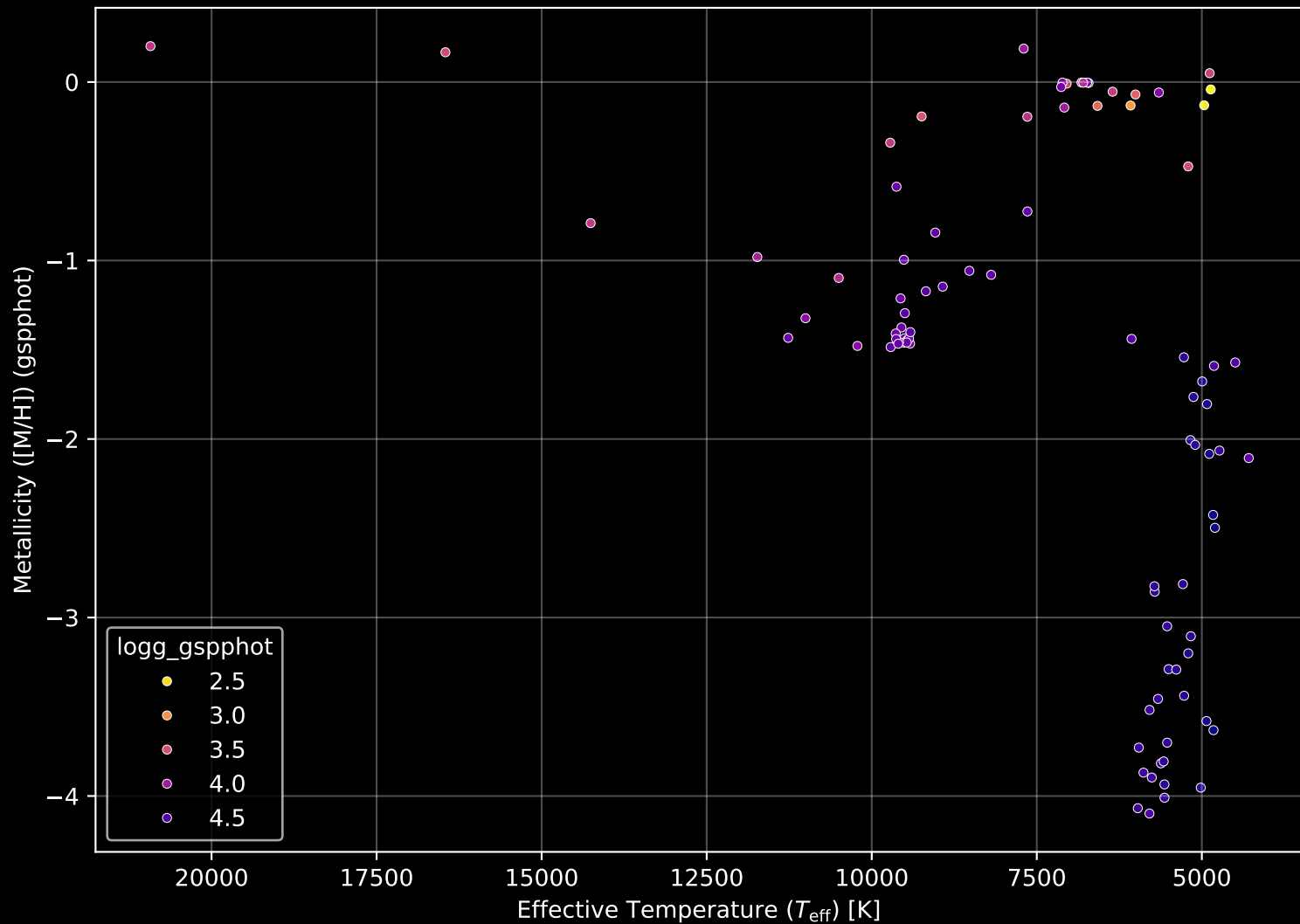
Gaia Cluster: [Teutsch_52] Stellar Population Parameters (n= 90)
