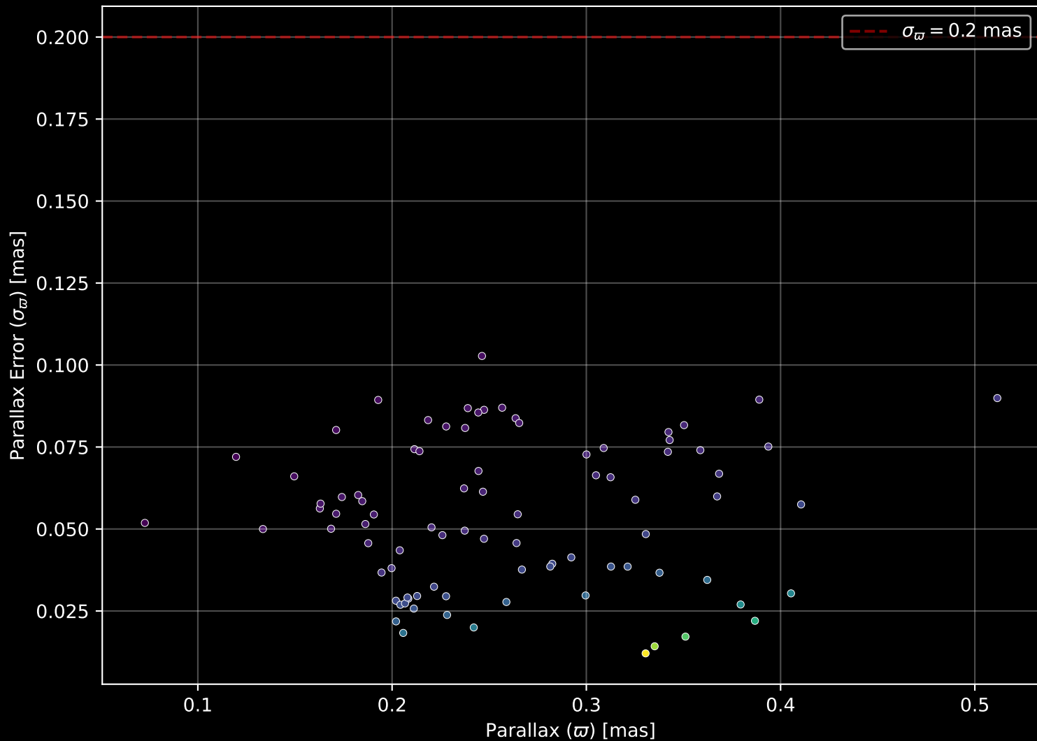
Gaia Cluster: [Deutsch_54] Parallax Quality (n= 86)
