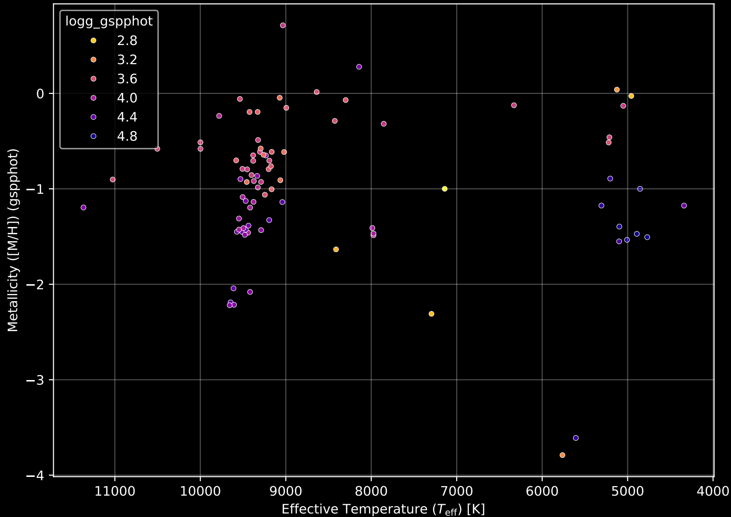
Gaia Cluster: [Deutsch_54] Stellar Population Parameters (n= 86)
