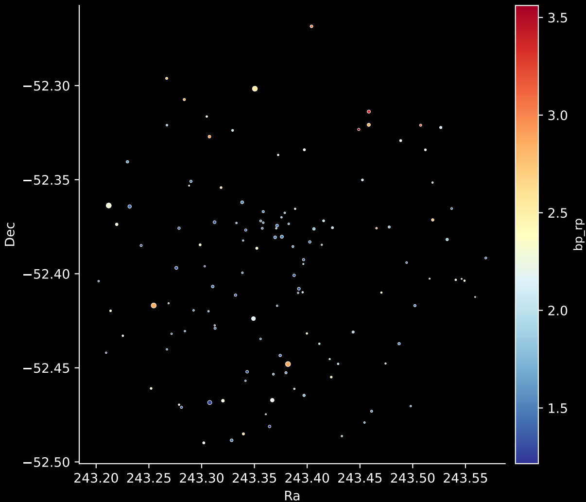
Gaia Cluster: [Deutsch_66] Stars: 125
