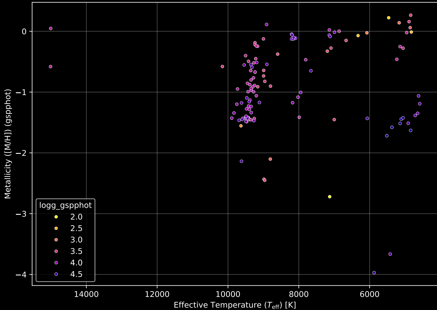
Gaia Cluster: [Teutsch_66] Stellar Population Parameters (n= 125)
