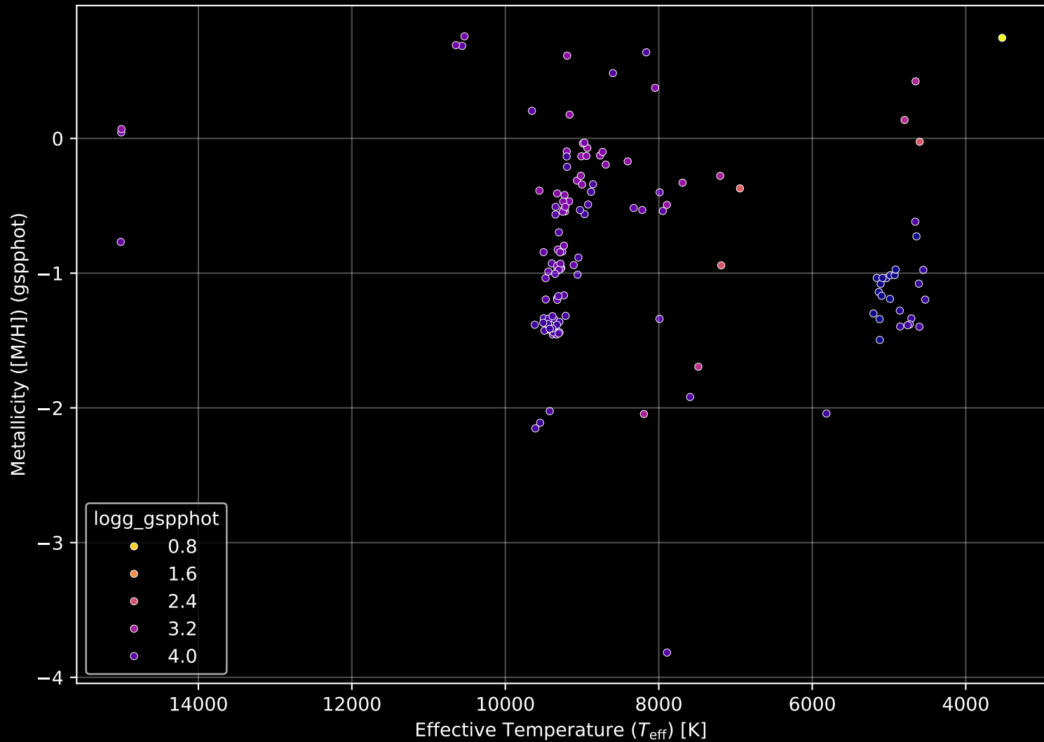
Gaia Cluster: [Deutsch_84] Stellar Population Parameters (n= 136)
