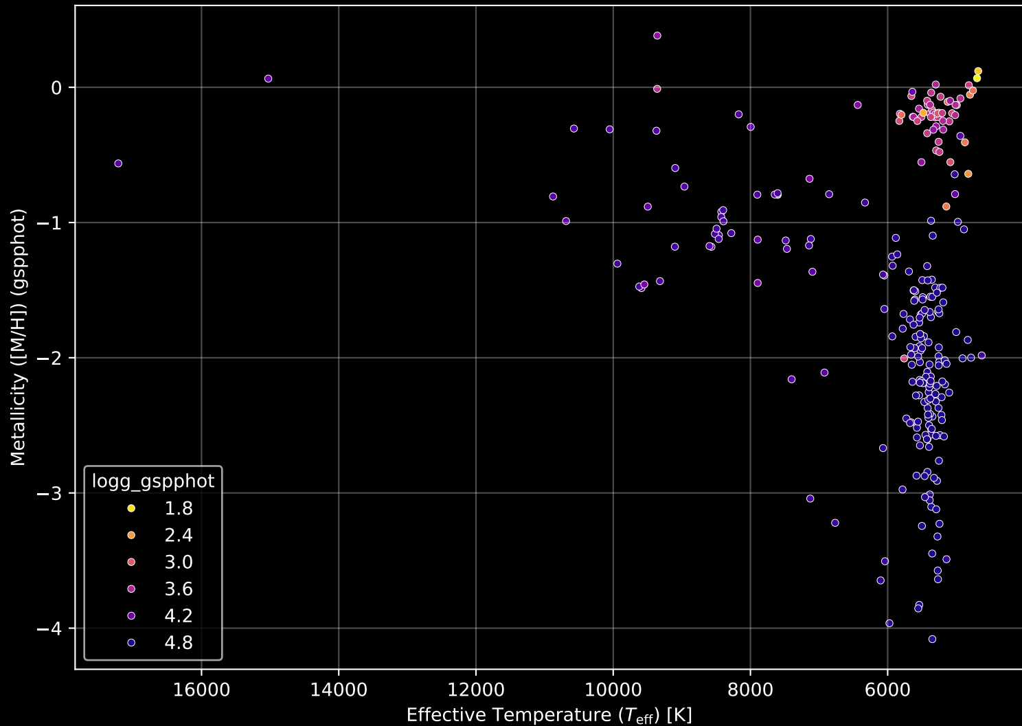
Gaia Cluster: [Tombaugh_2] Stellar Population Parameters (n= 260)
