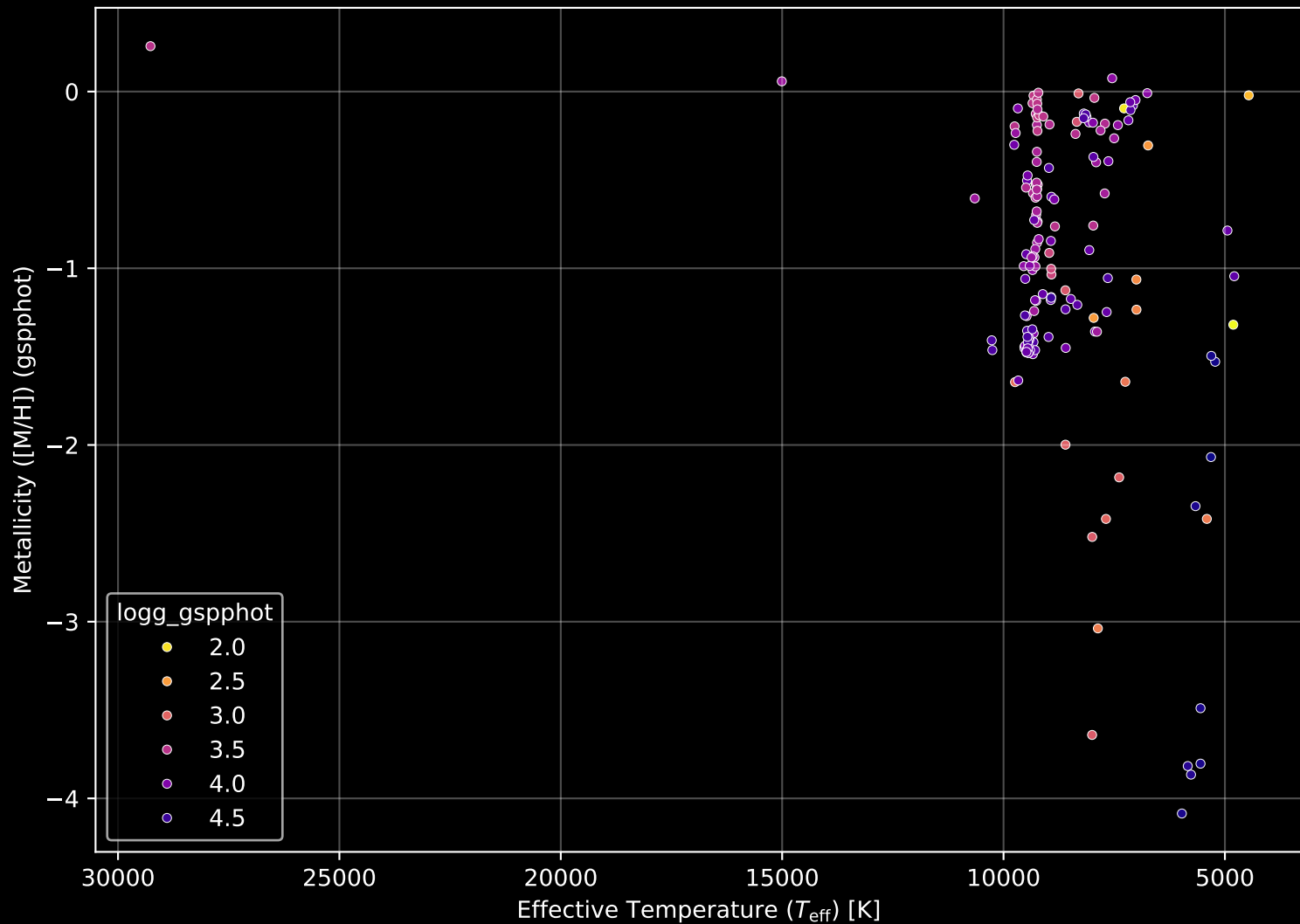
Gaia Cluster: [Tombaugh_4] Stellar Population Parameters (n= 160)
