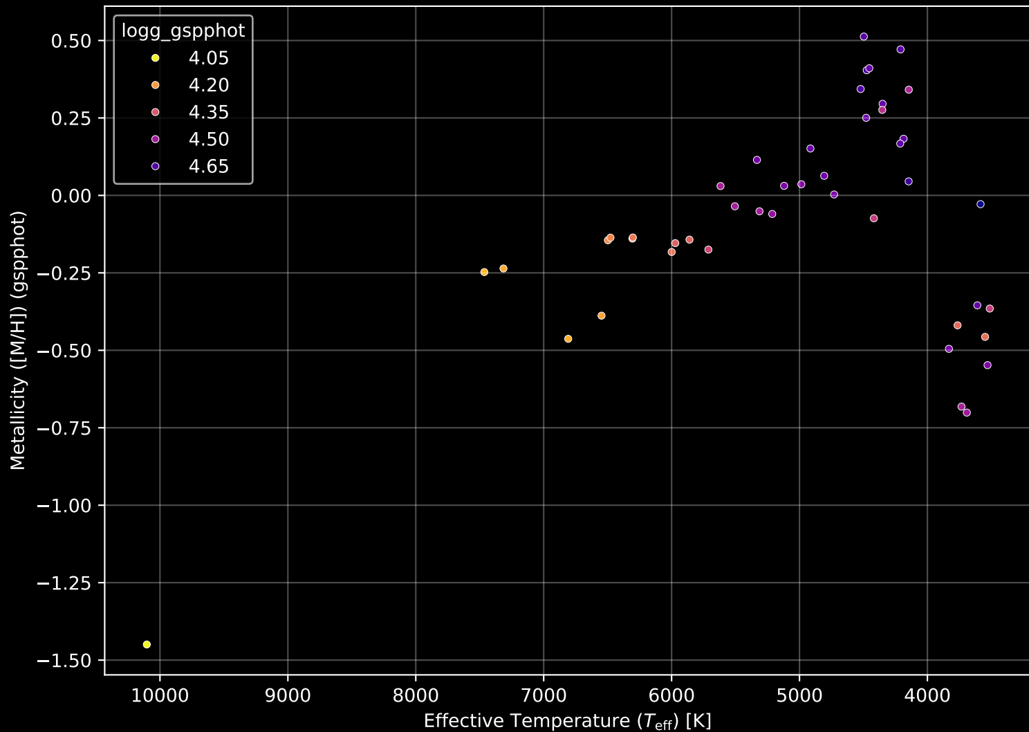
Gaia Cluster: [UBC_1] Stellar Population Parameters (n= 45)
