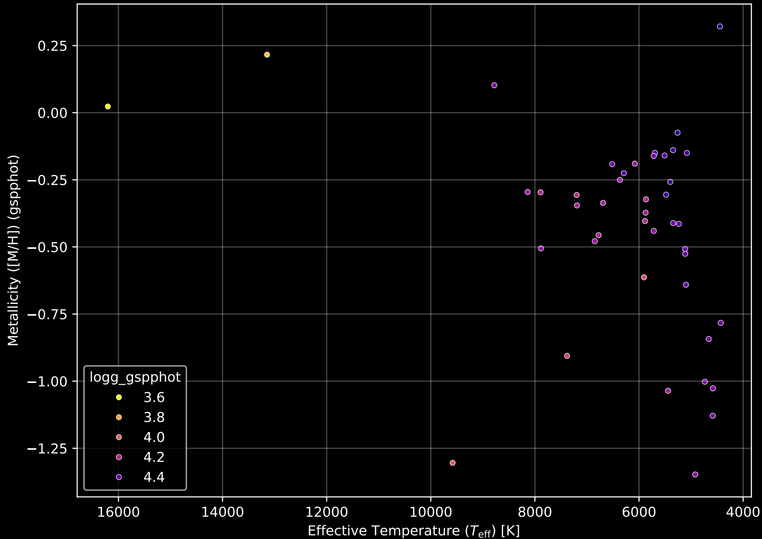
Gaia Cluster: [UBC_14] Stellar Population Parameters (n= 43)
