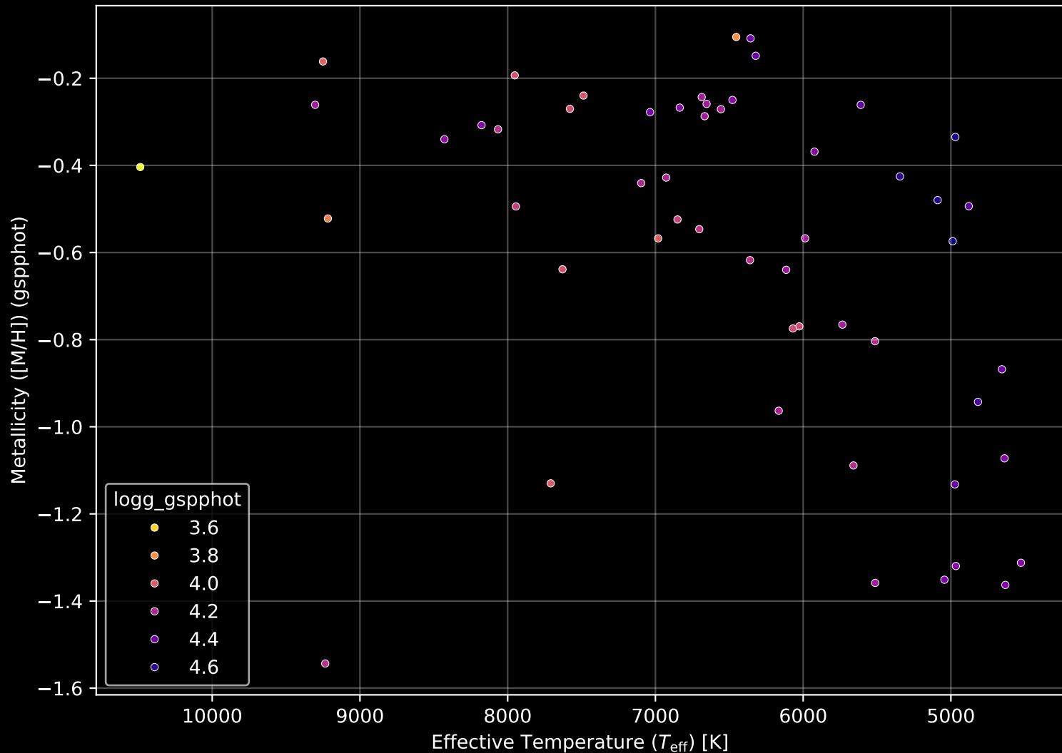
Gaia Cluster: [UBC_27] Stellar Population Parameters (n= 54)
