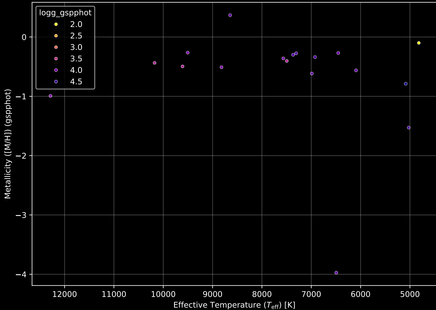
Gaia Cluster: [UBC_3] Stellar Population Parameters (n= 18)
