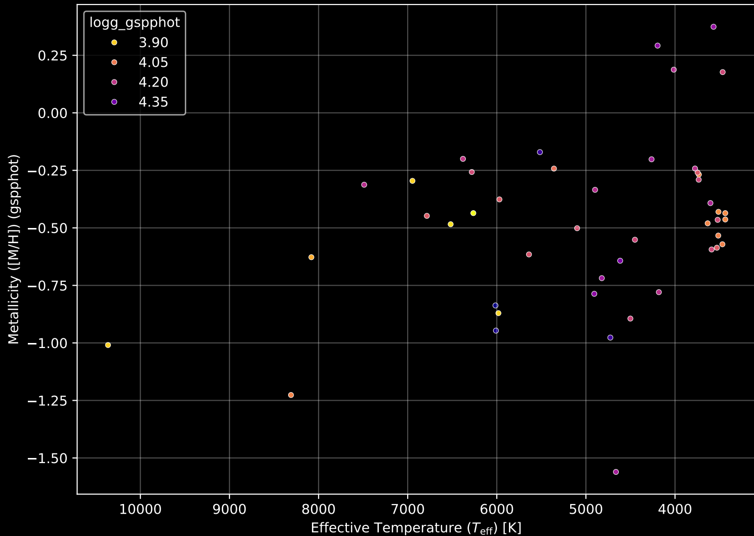
Gaia Cluster: [UBC_31] Stellar Population Parameters (n= 46)
