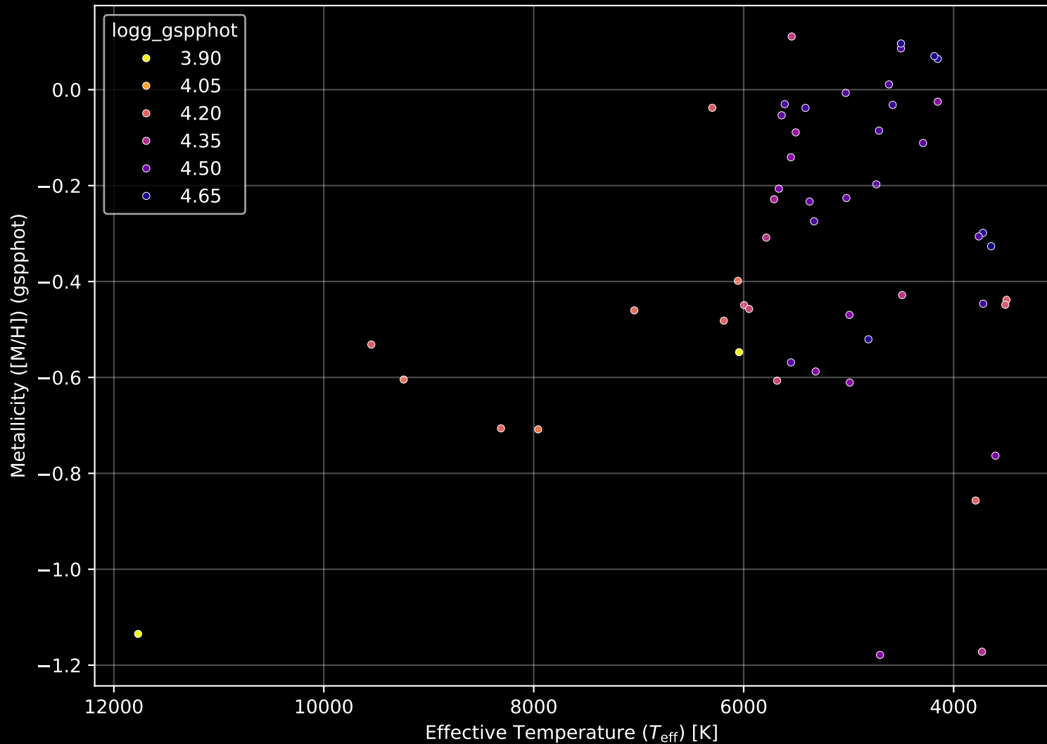
Gaia Cluster: [UBC_32] Stellar Population Parameters (n= 52)
