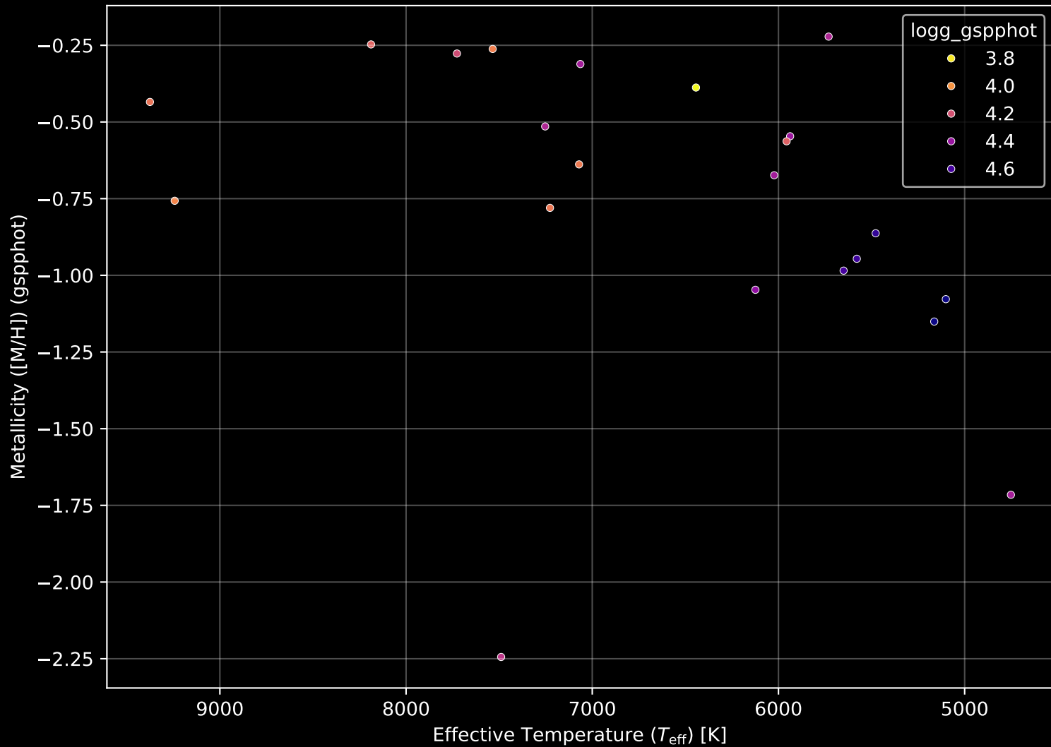
Gaia Cluster: [UBC_36] Stellar Population Parameters (n= 22)
