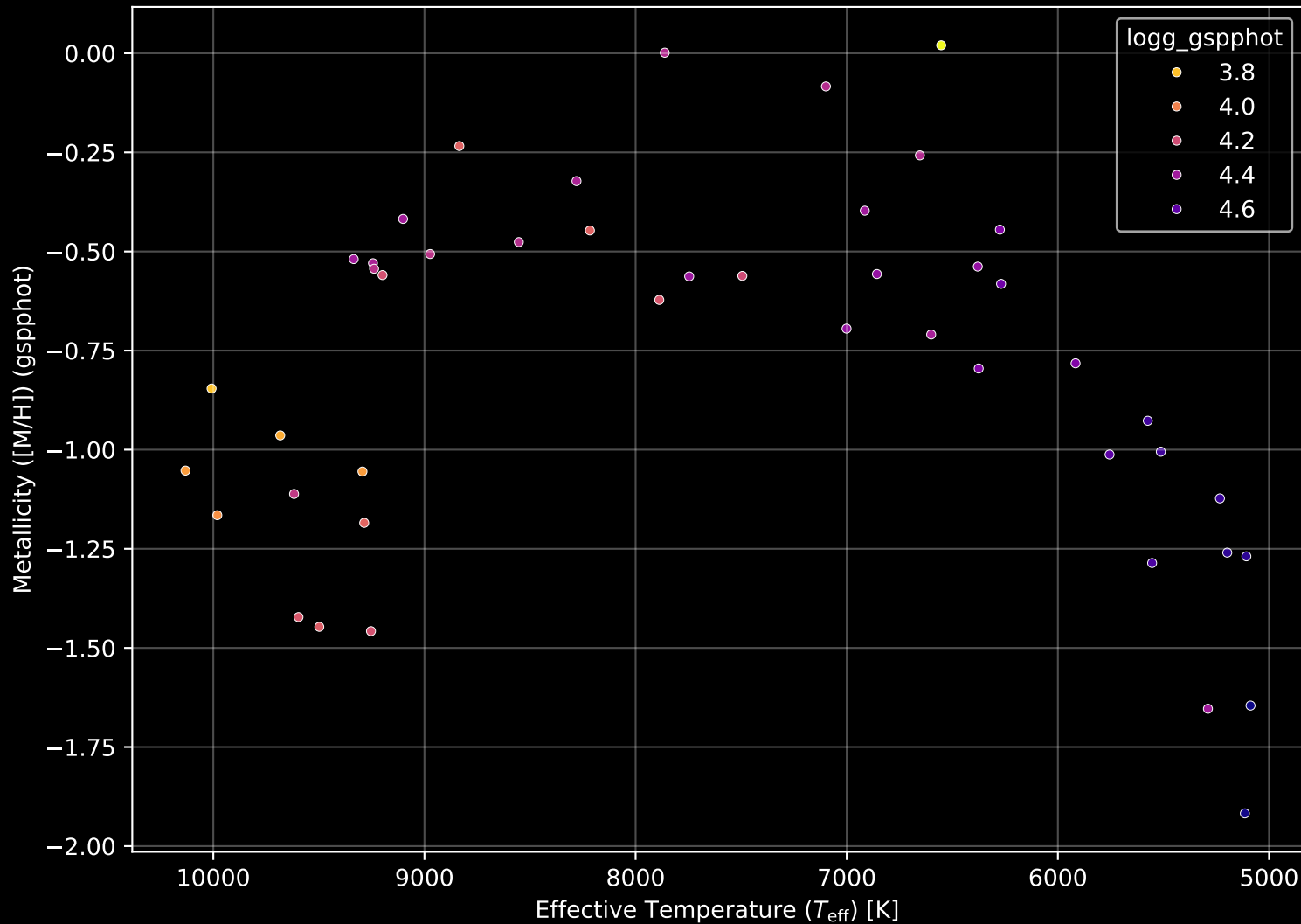
Gaia Cluster: [UBC_73] Stellar Population Parameters (n= 46)
