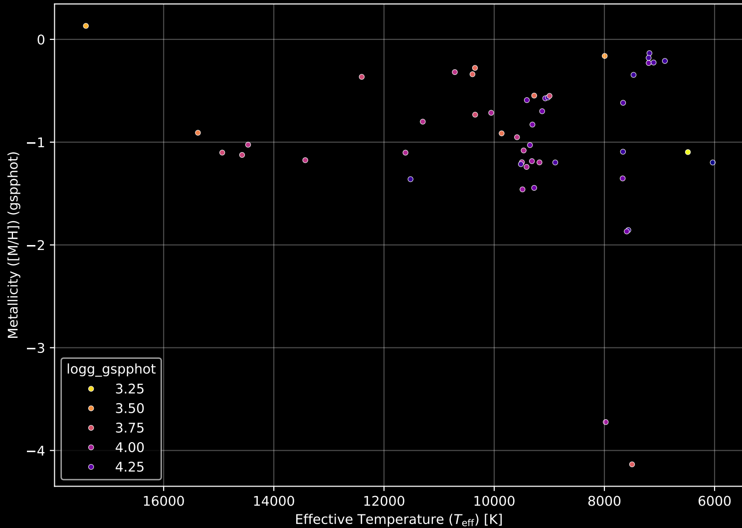
Gaia Cluster: [UBC_84] Stellar Population Parameters (n= 50)
