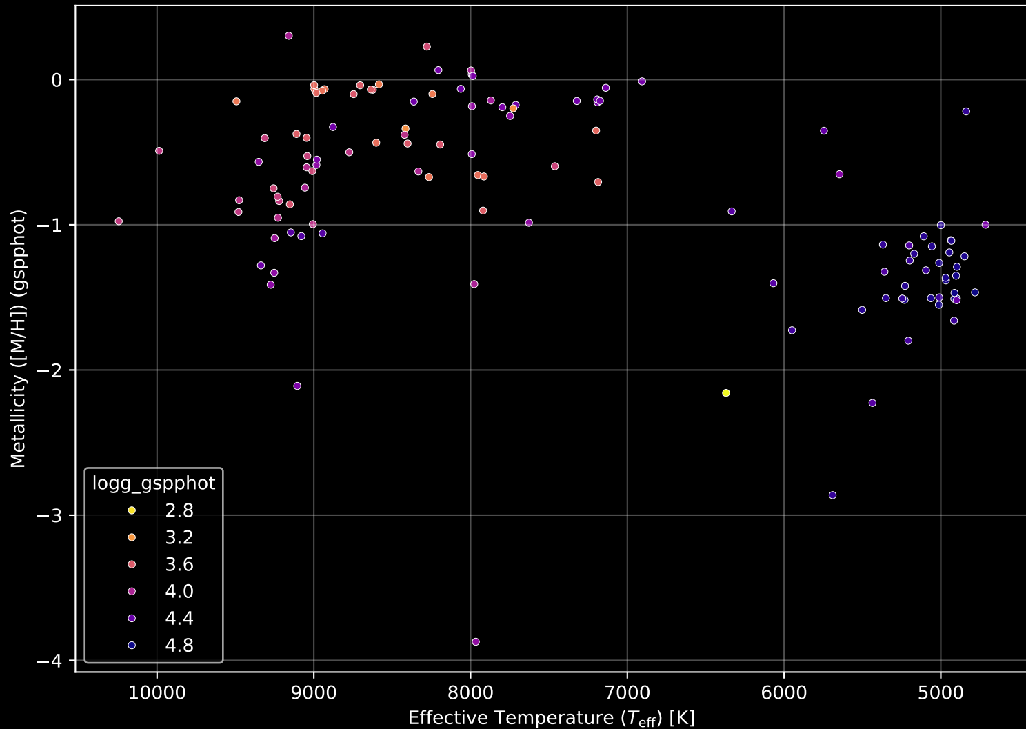
Gaia Cluster: [UFMG_1] Stellar Population Parameters (n= 122)
