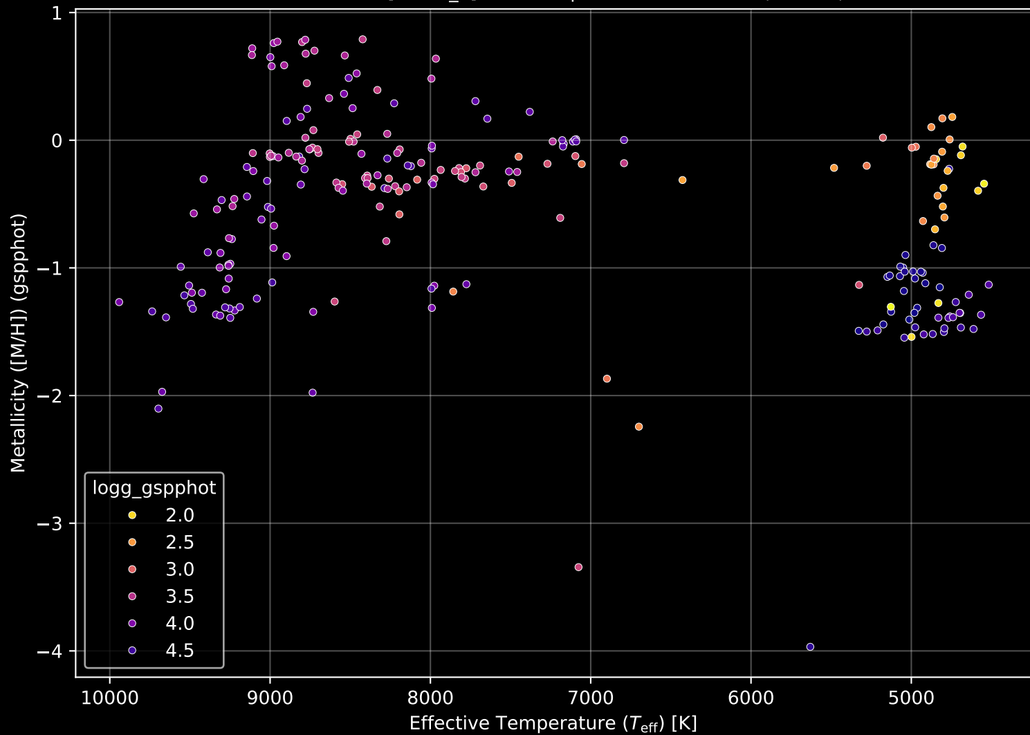
Gaia Cluster: [UFMG_2] Stellar Population Parameters (n= 247)
