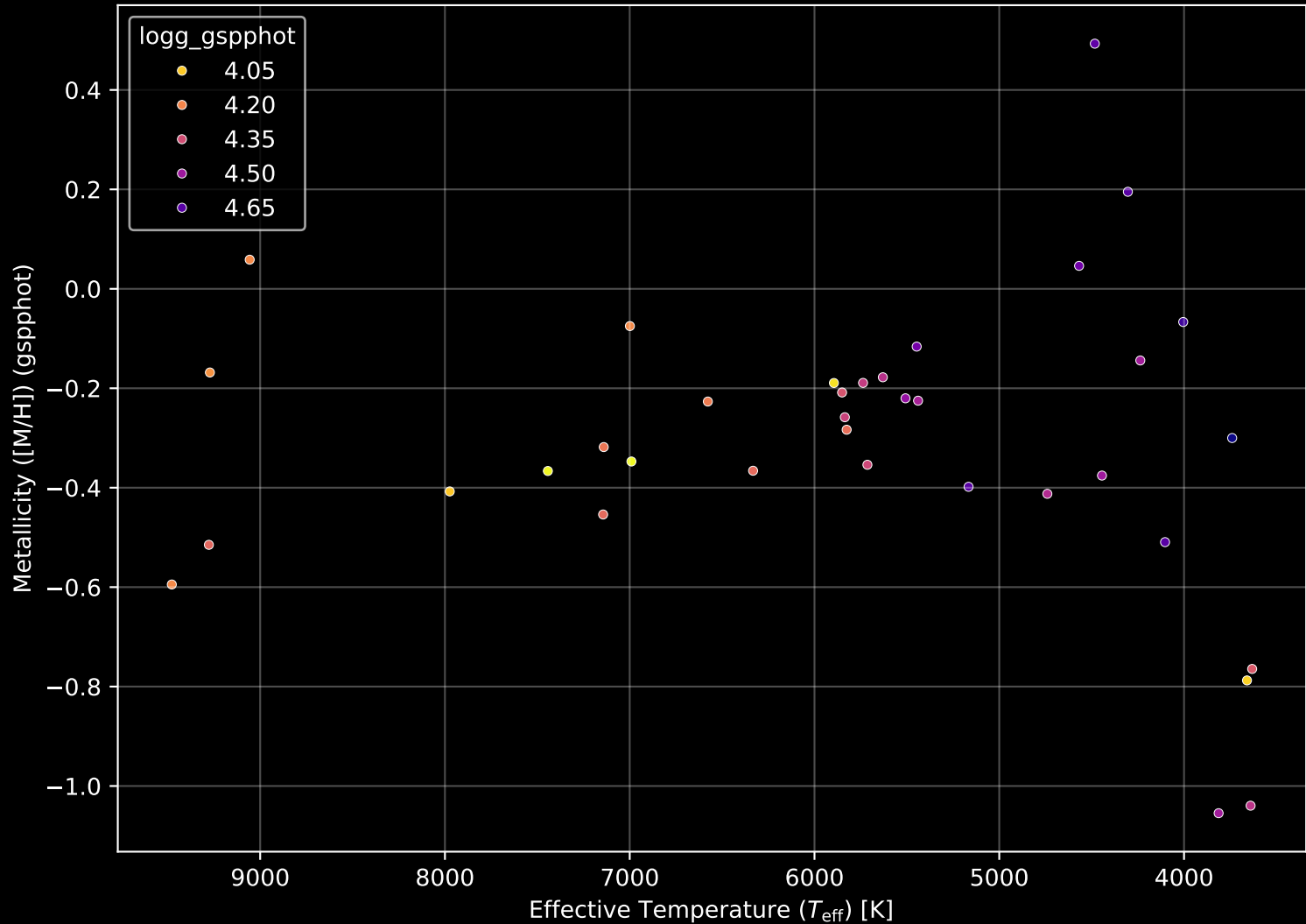
Gaia Cluster: [UPK_137] Stellar Population Parameters (n= 36)
