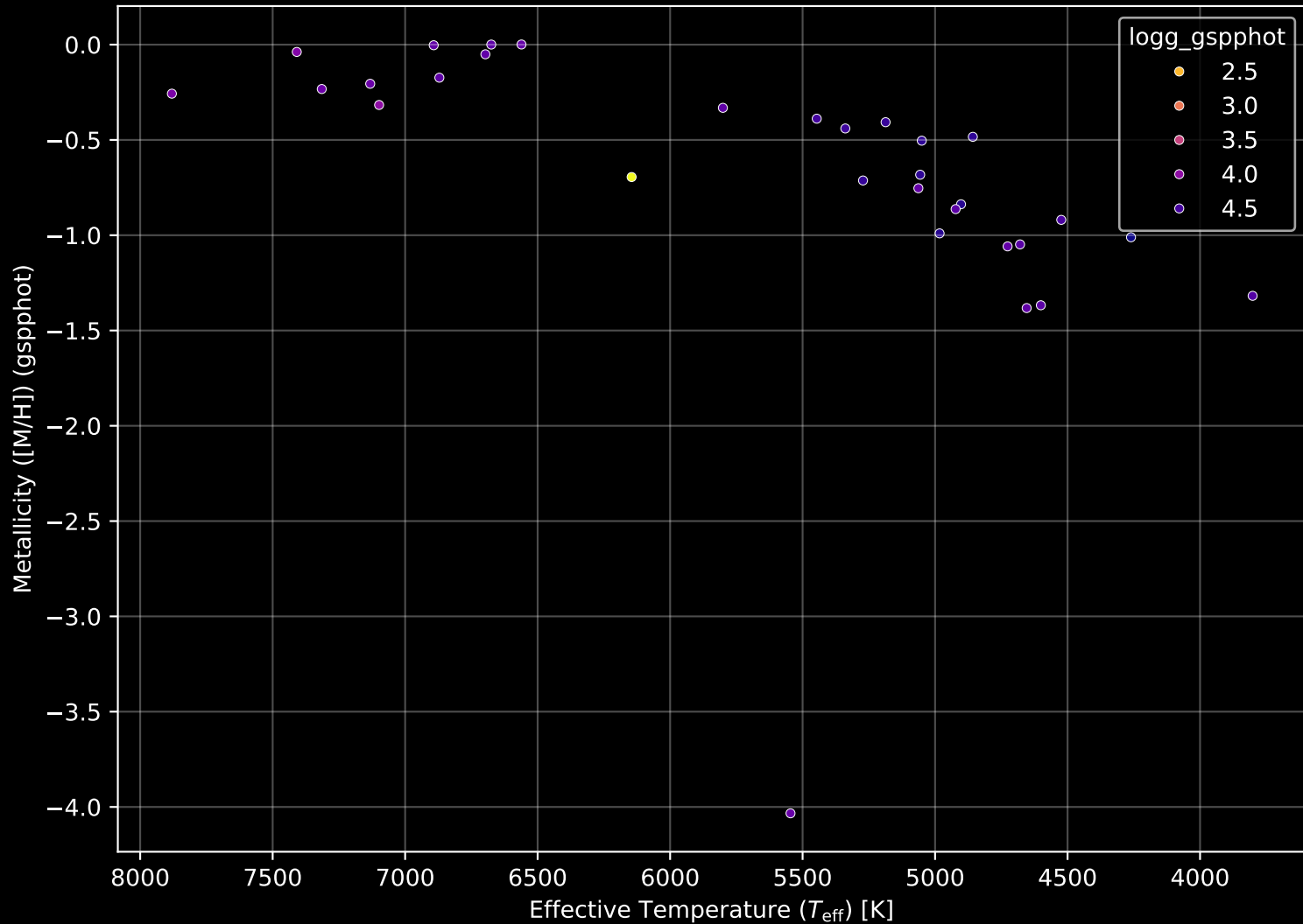
Gaia Cluster: [UPK_178] Stellar Population Parameters (n= 31)
