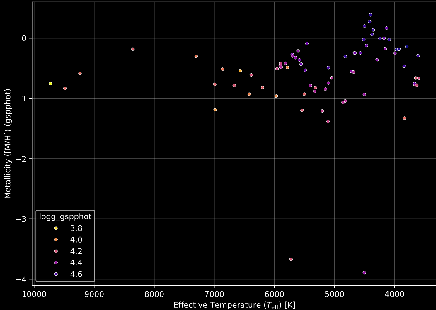
Gaia Cluster: [UPK_20] Stellar Population Parameters (n= 76)
