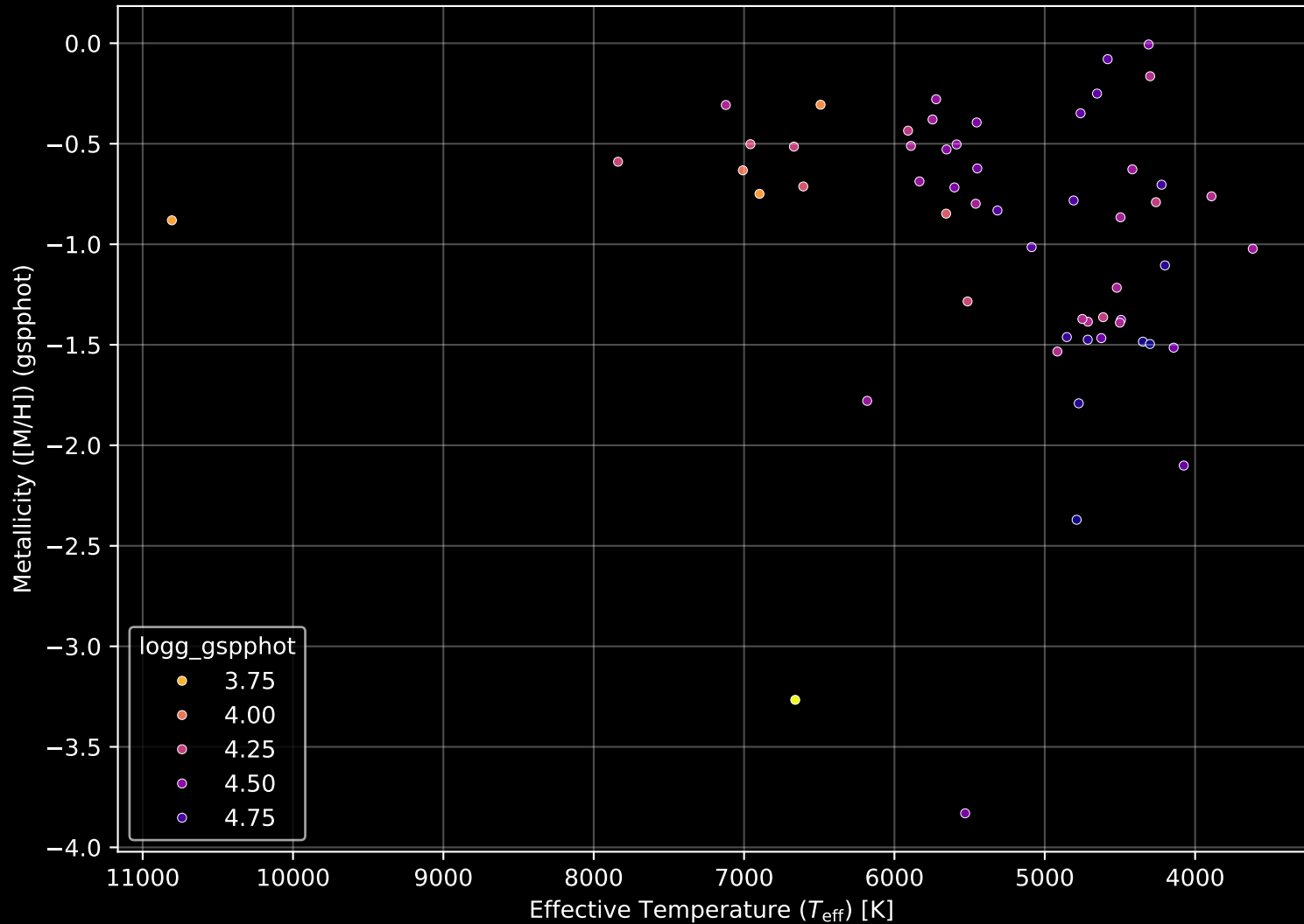
Gaia Cluster: [UPK_23] Stellar Population Parameters (n= 56)
