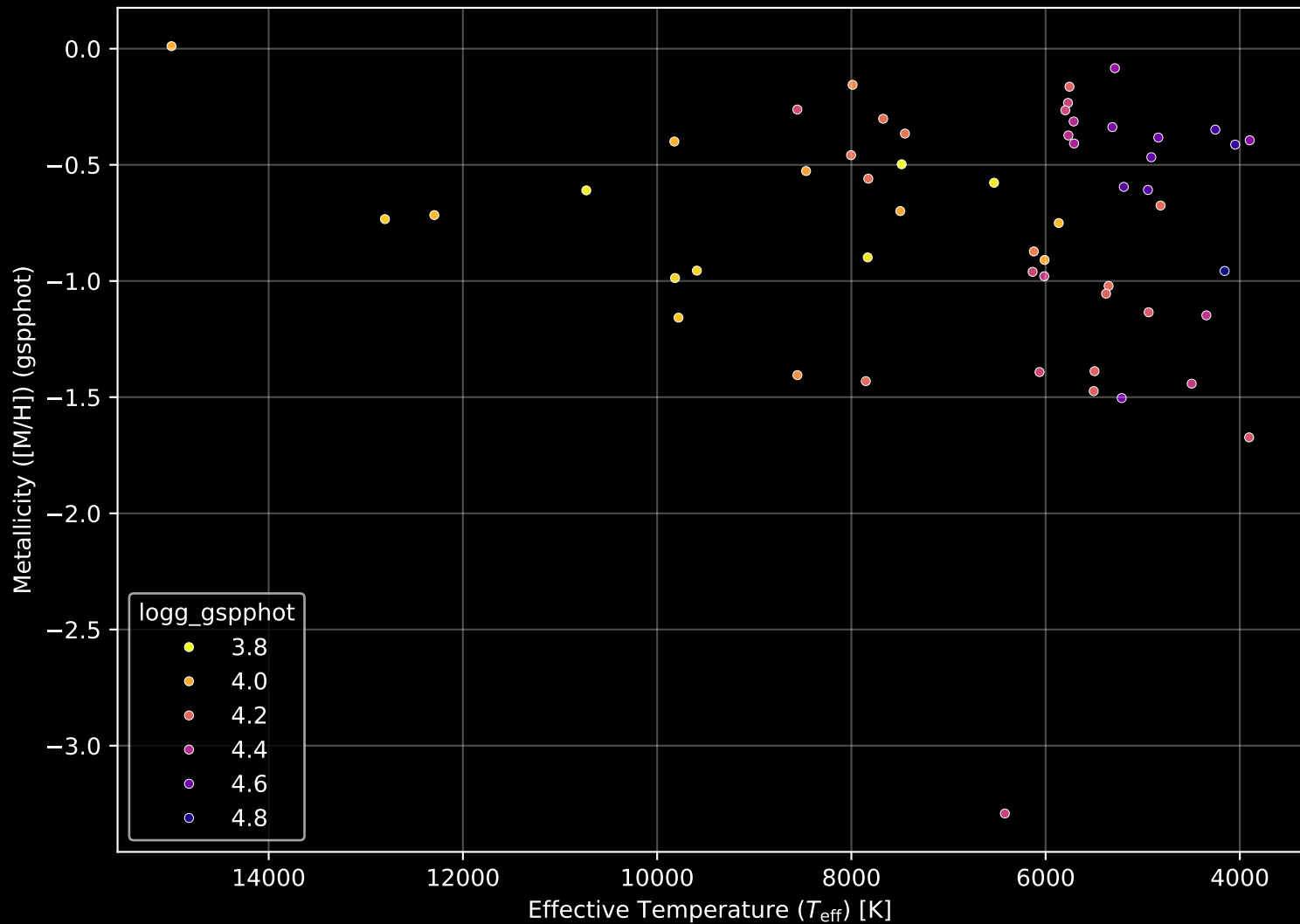
Gaia Cluster: [UPK_28] Stellar Population Parameters (n= 54)
