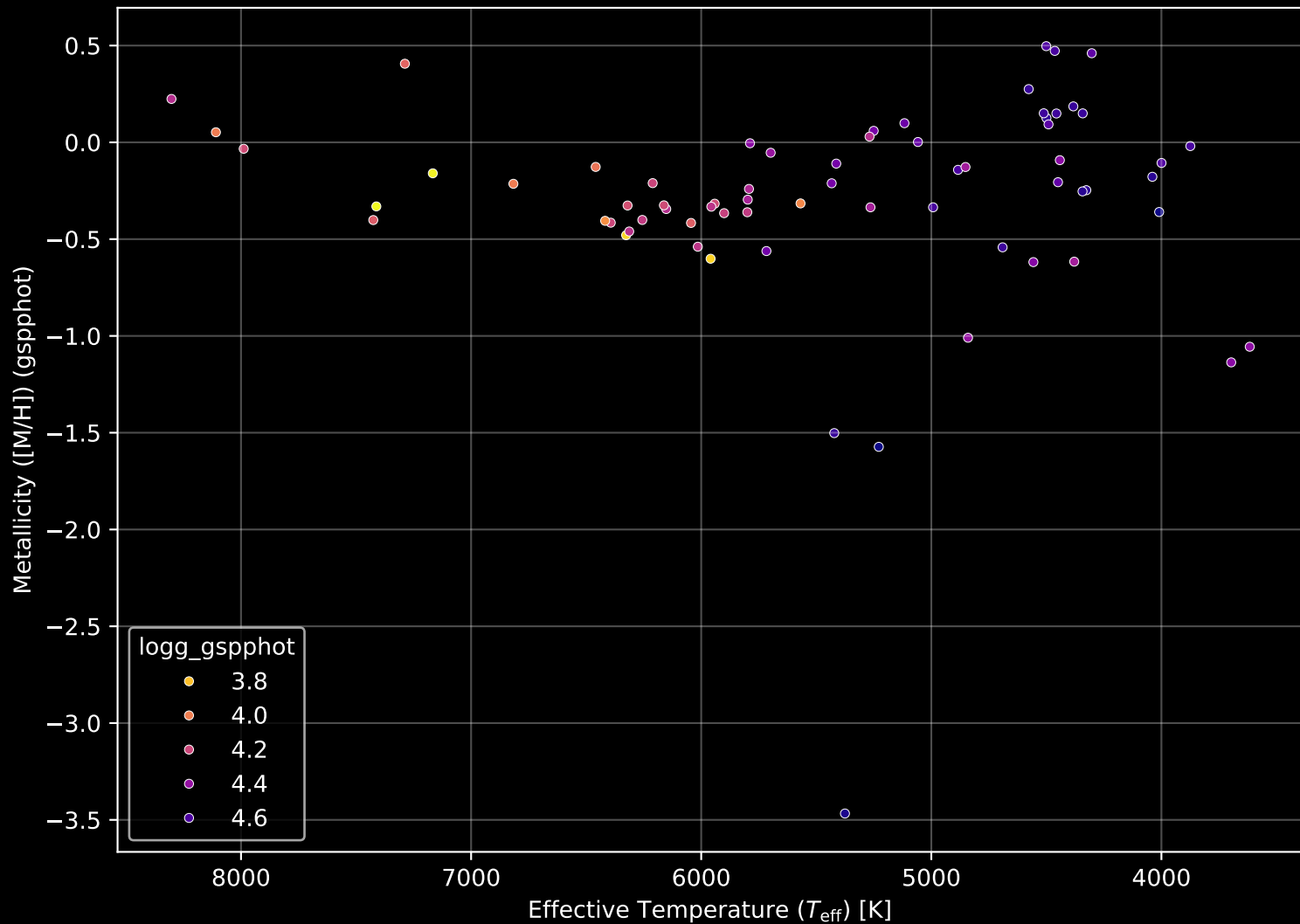
Gaia Cluster: [UPK_294] Stellar Population Parameters (n= 68)
