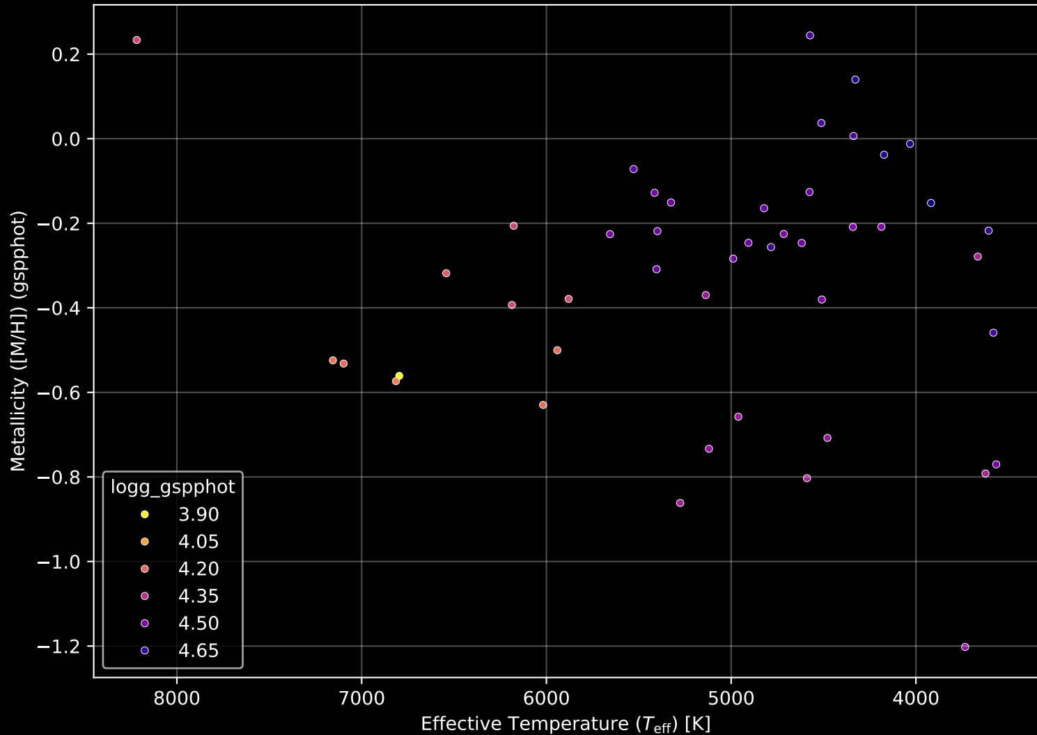
Gaia Cluster: [UPK_31] Stellar Population Parameters (n= 46)
