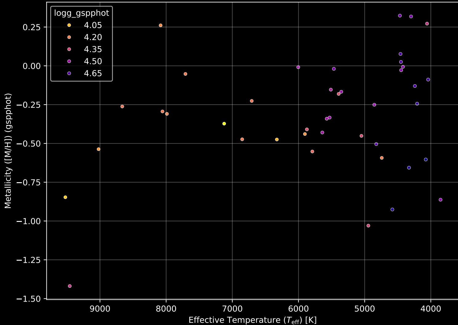
Gaia Cluster: [UPK_312] Stellar Population Parameters (n= 42)
