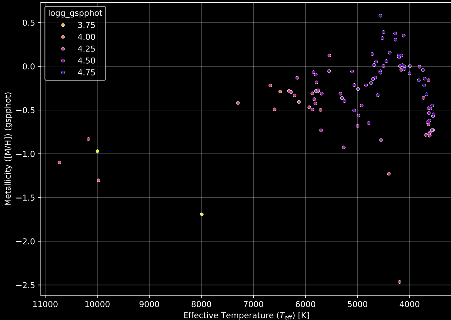
Gaia Cluster: [UPK_524] Stellar Population Parameters (n= 97)
